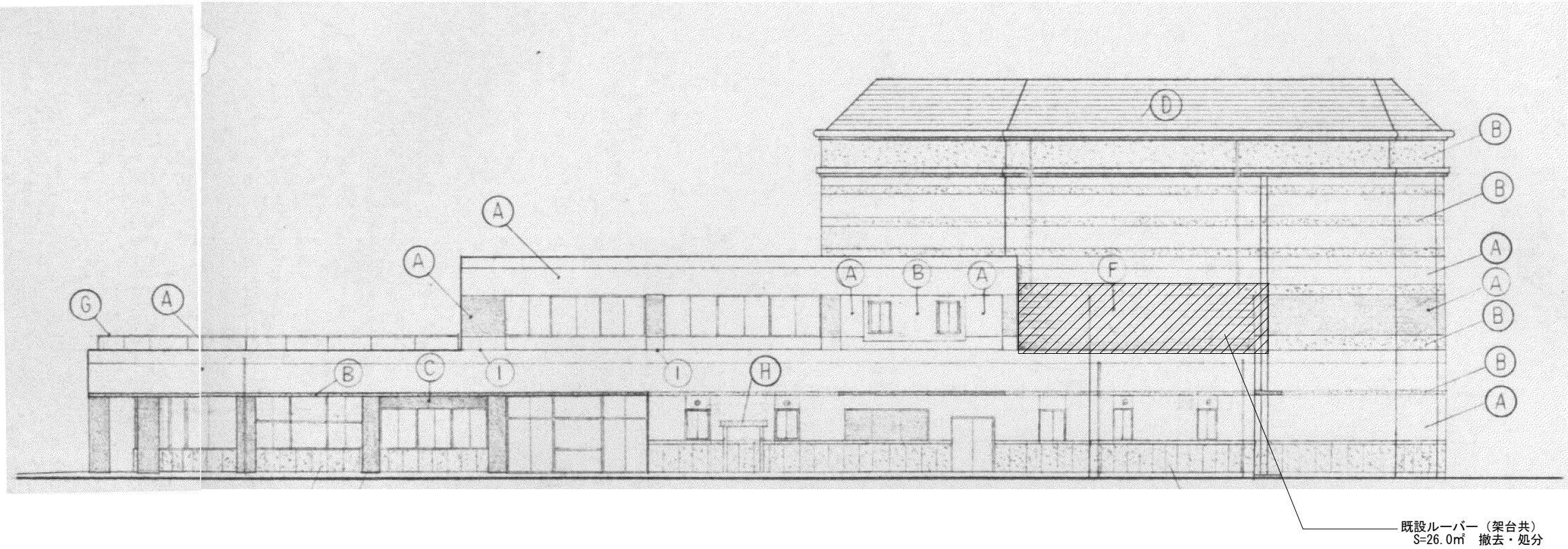
東立面図 S = 1 / 2 0 0
