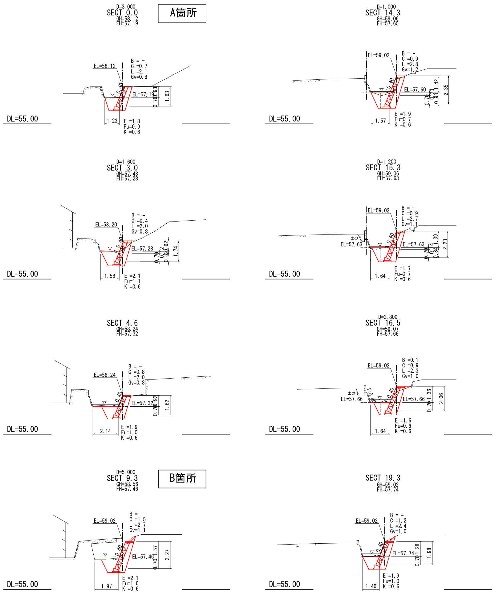
横断面図 縮尺=1:100
