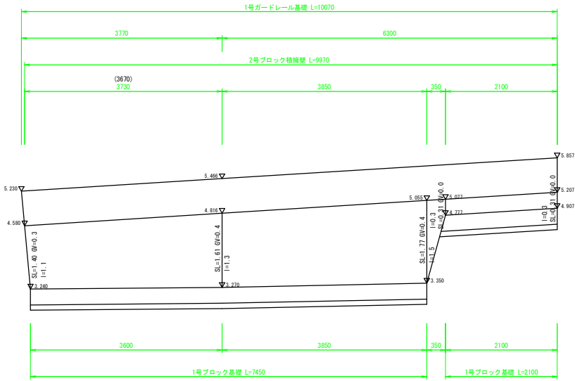
2号ブロック積擁壁展開図 S=1:50
