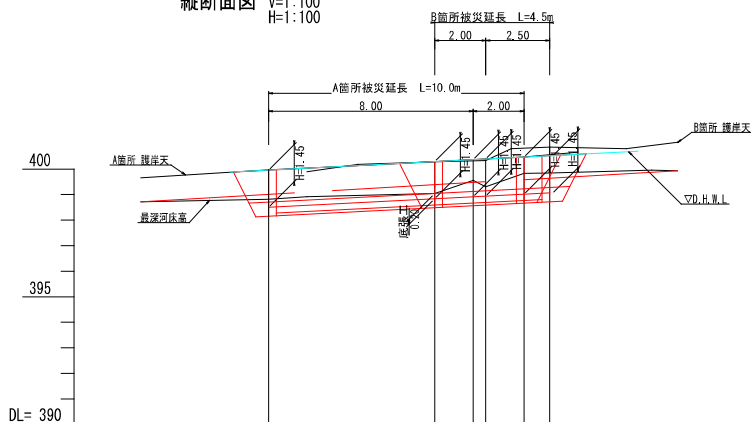
縦断面図 V=1:100 H=1:100
