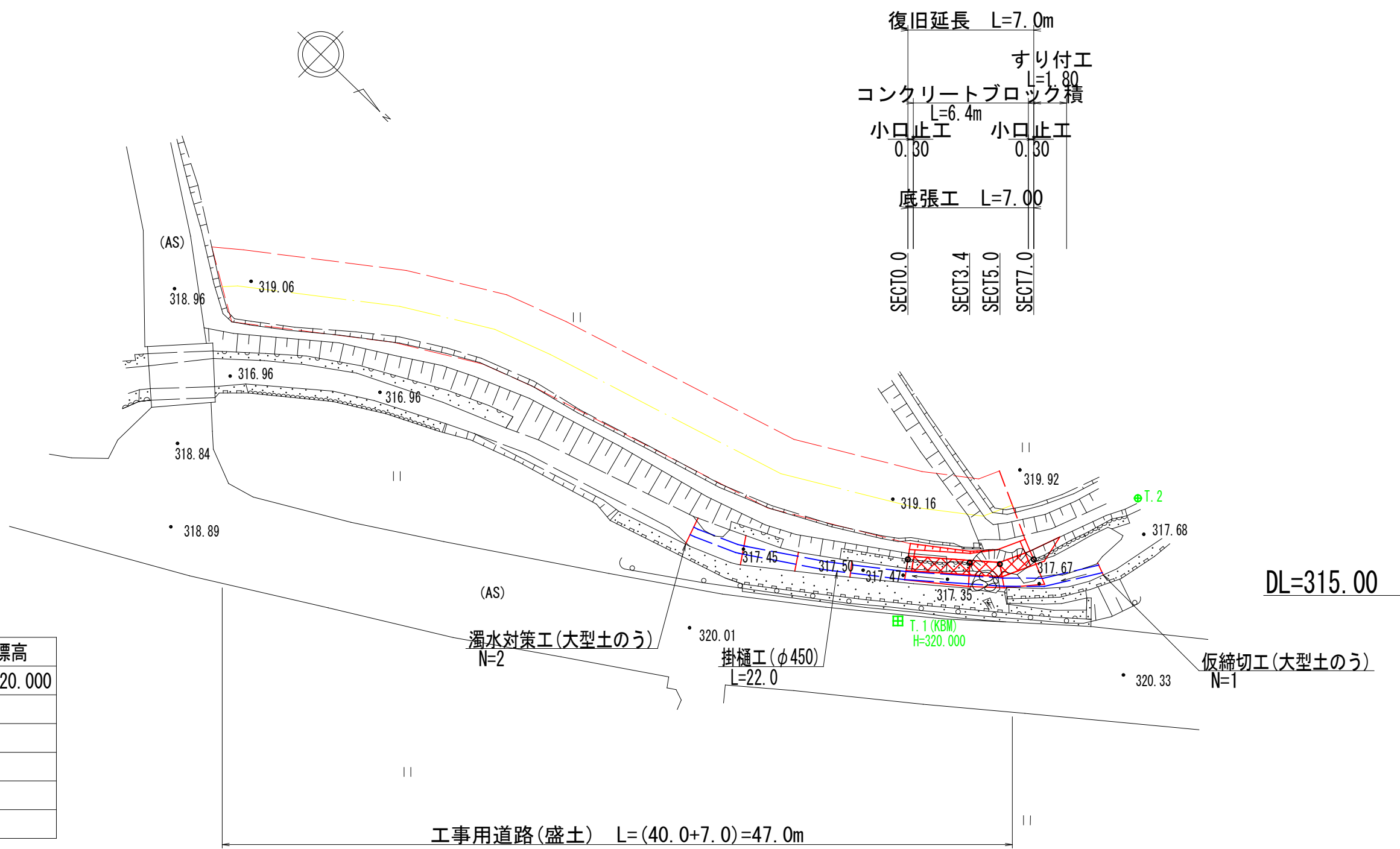
平 面 図 S=1:250
