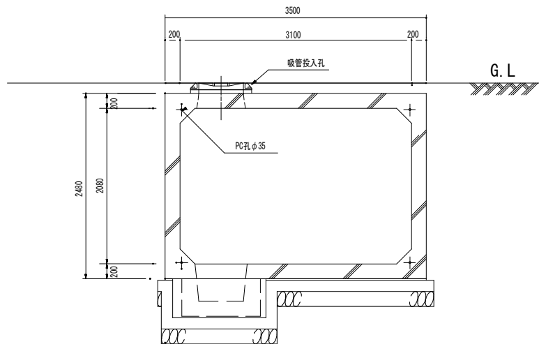
断面図 1/50
