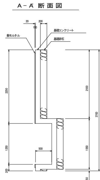
A-A 断面図
