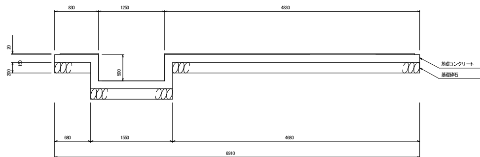
C-C 断面図
