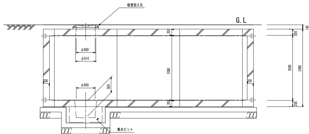
断面図 1/50
