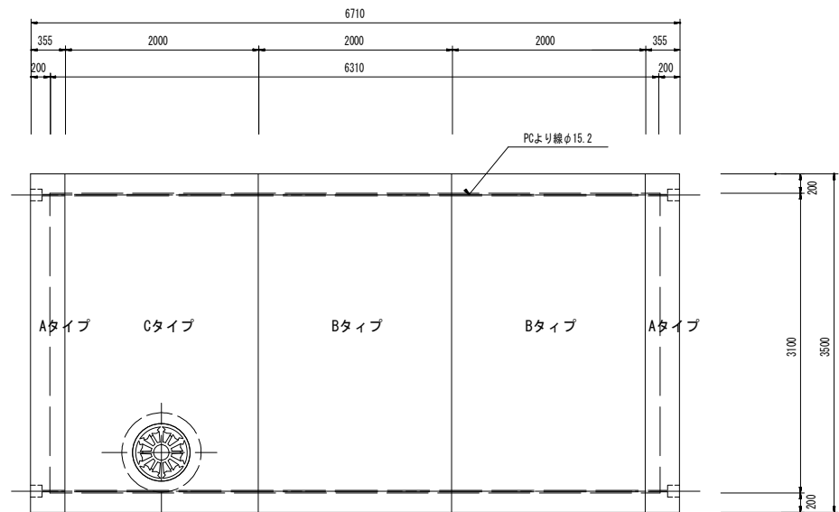
平面図 1/50
