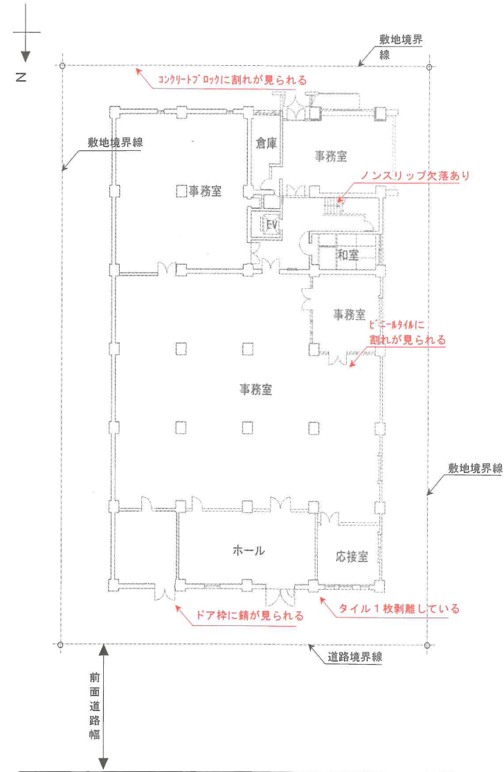
配置図兼1階平面図 S:1 1/400
