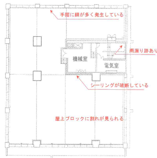
屋上平面図 S:1 1/400
