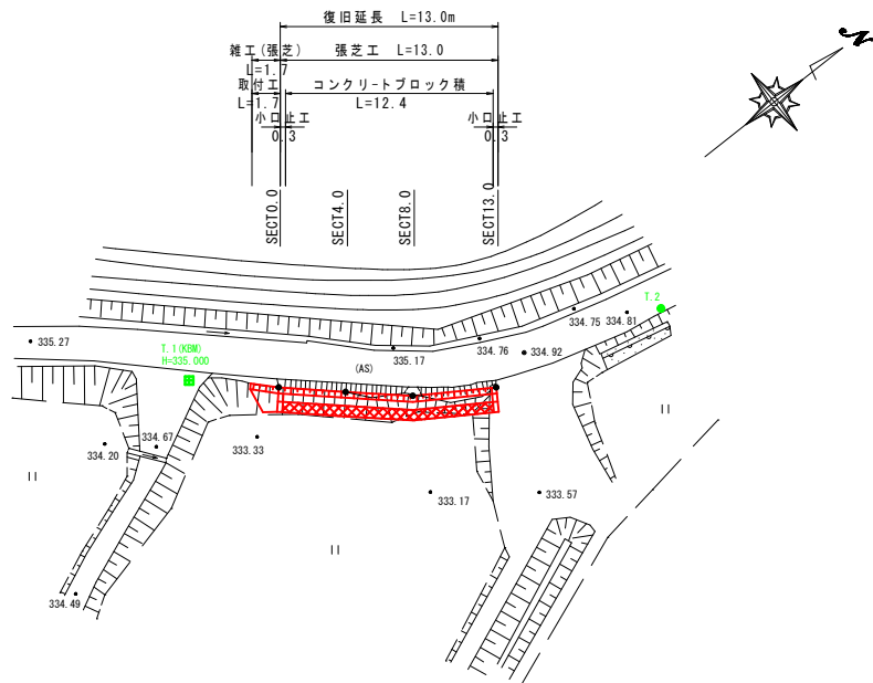
平面図 S=1:250
