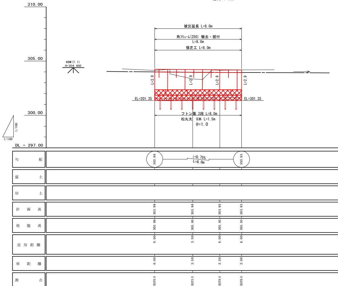
縦断面図 縮尺=1:100
