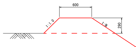
畦畔築立 縮尺=1:20
