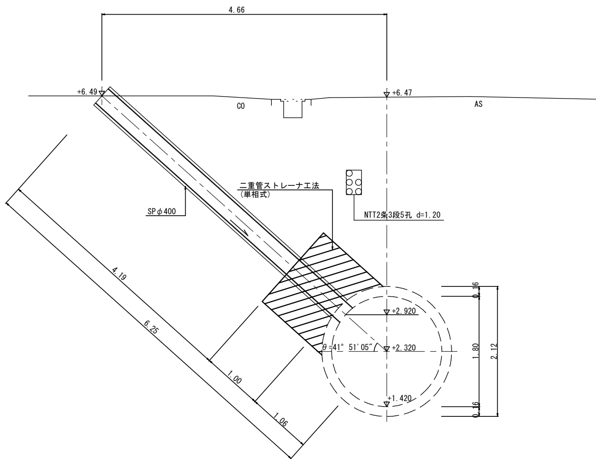
A-A断面図
