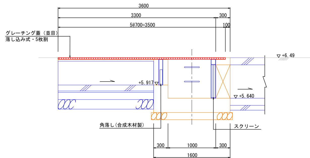
A-A断面
