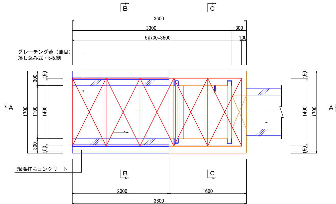
平面図
