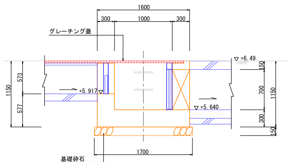
A-A断面
