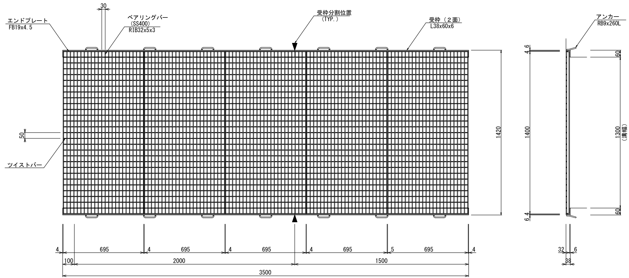
グレーチング蓋詳細図
