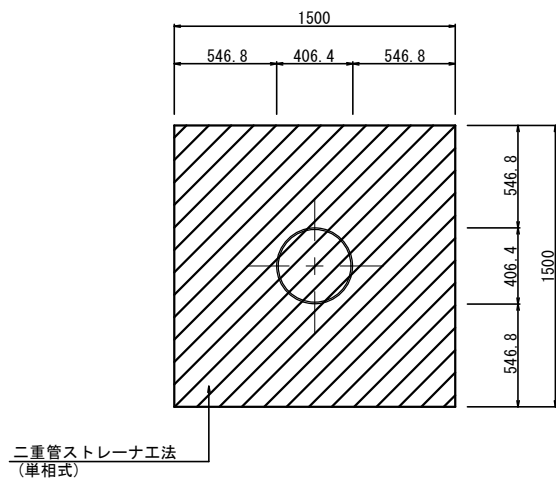
管路部断面図 S=1:20
