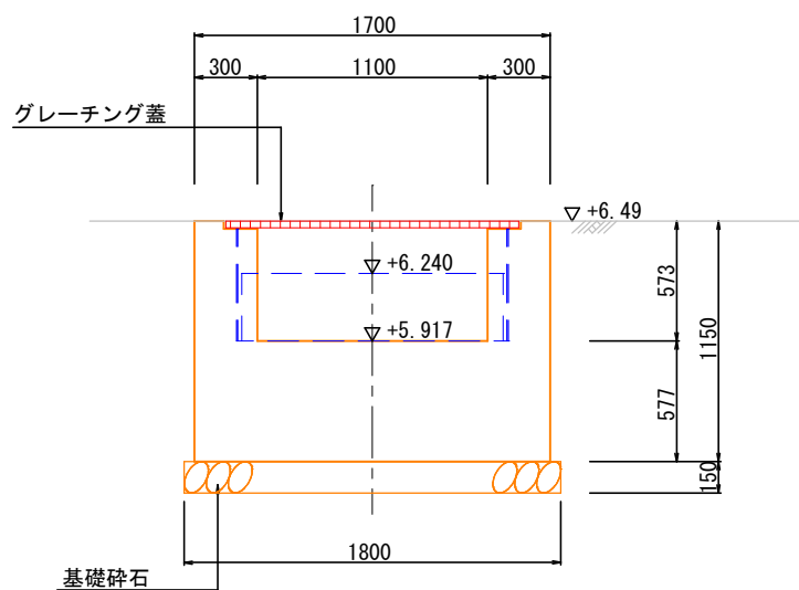
C-C断面
