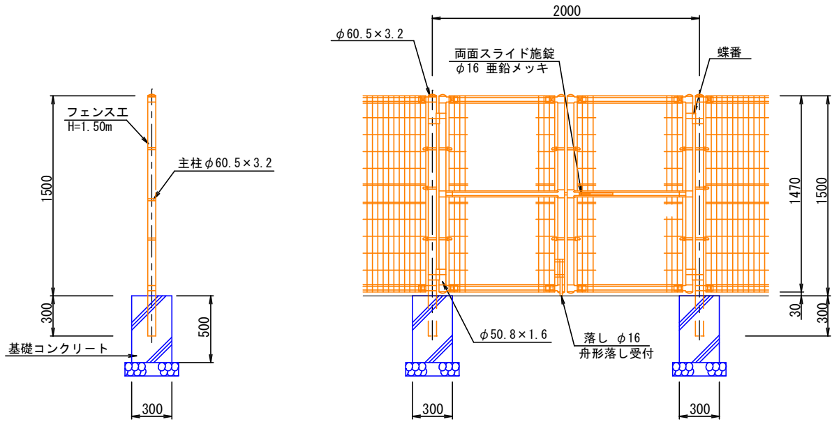
フェンス門扉工標準図 S=1:20
