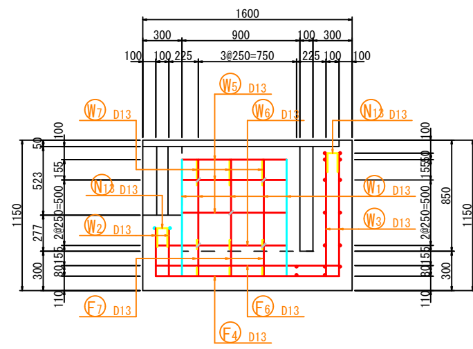
I - I (側壁内面)
