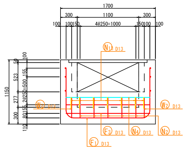
M - M (妻壁内面)
