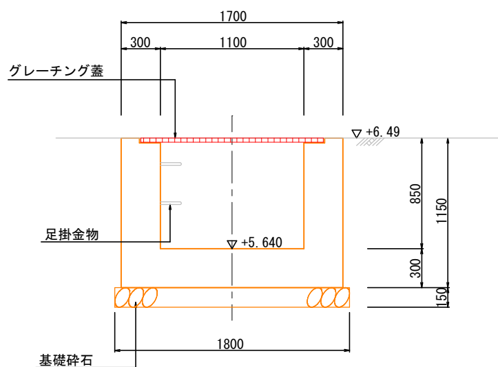
B-B断面
