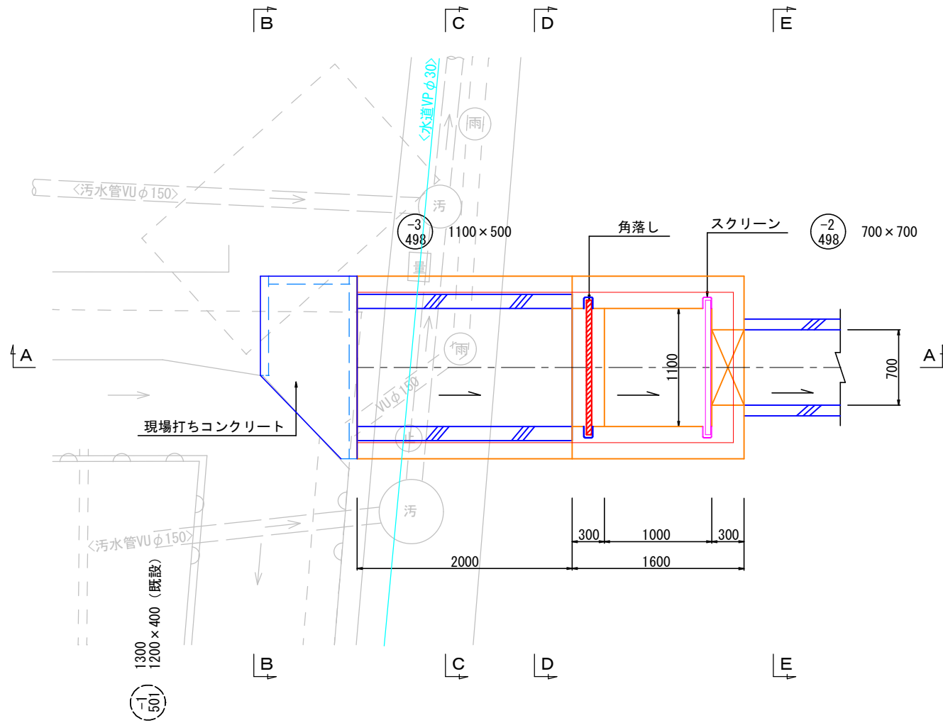
平面図
