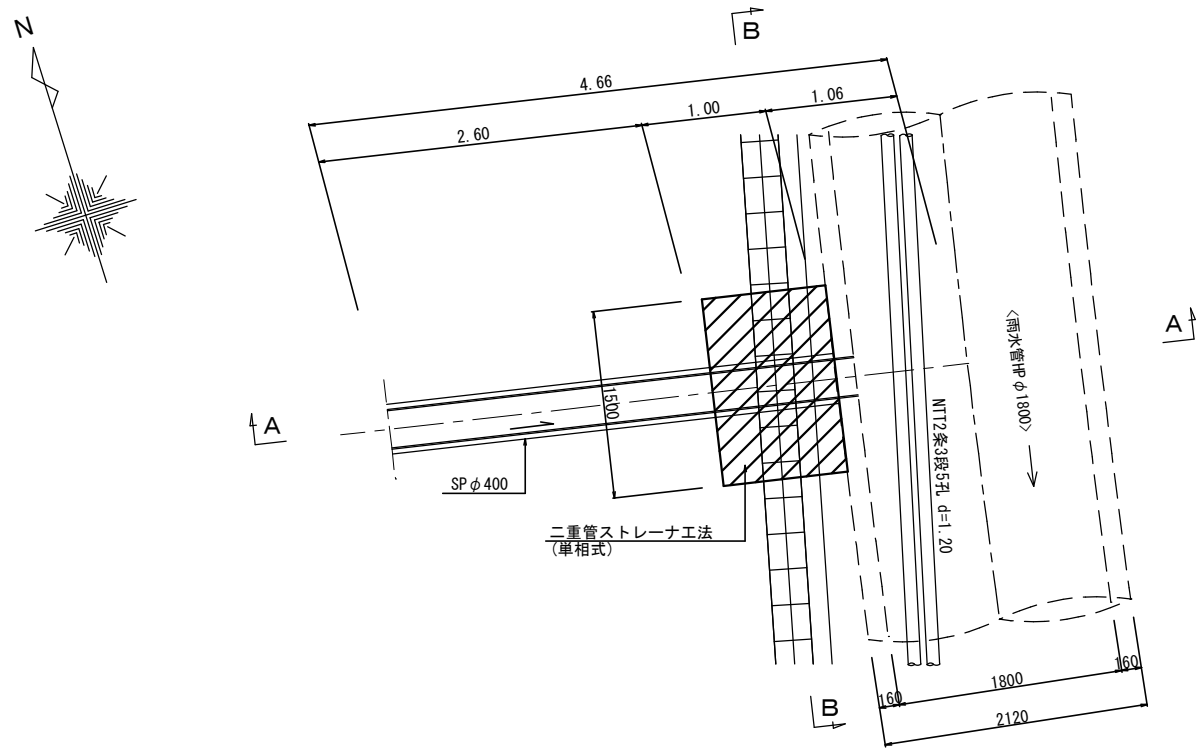
平面図
