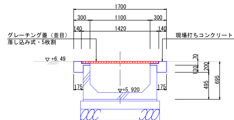
B-B断面
