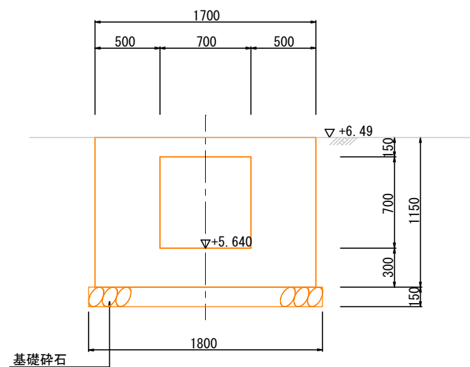
D-D断面
