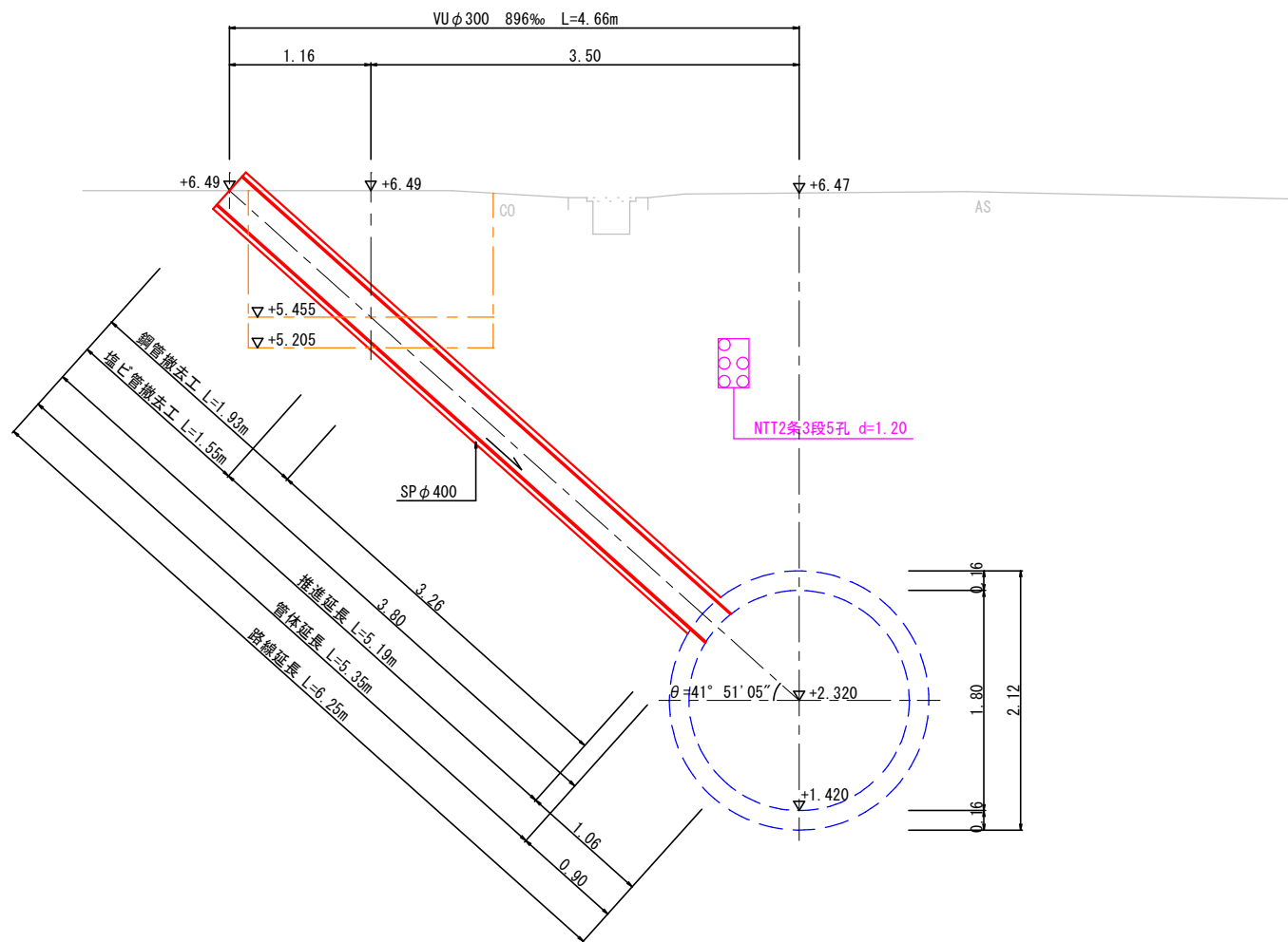
断面図
