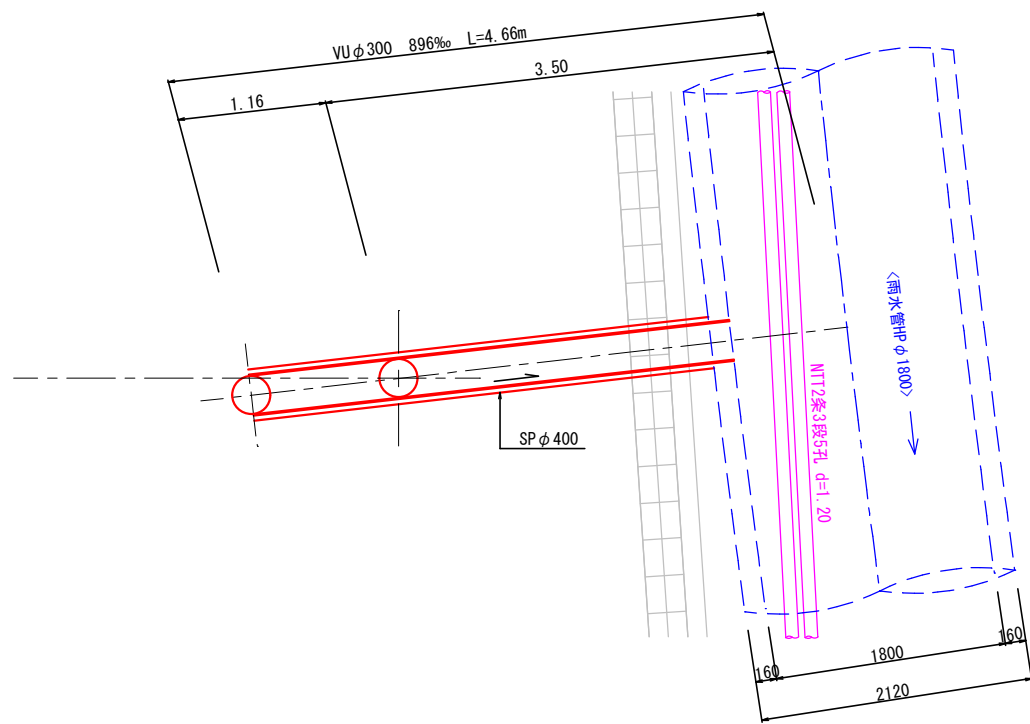
断面図
