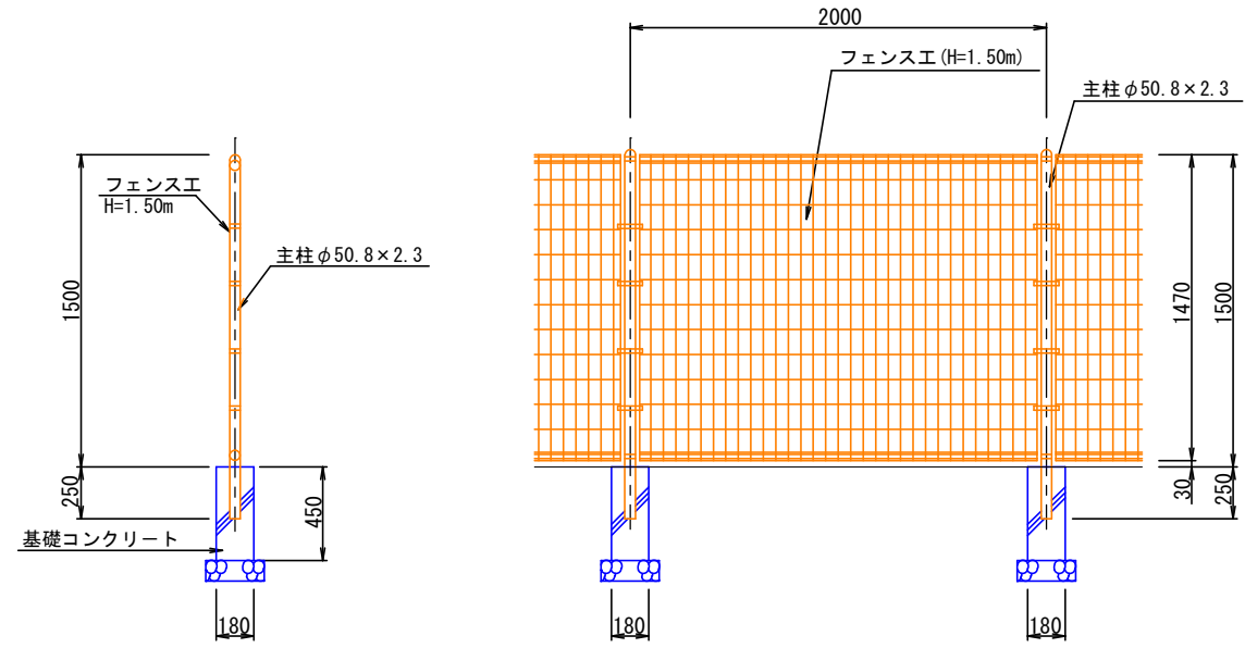
フェンス工標準図 S=1:20
