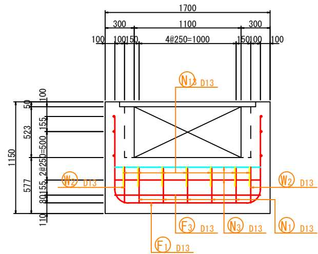
L - L (妻壁外面)
