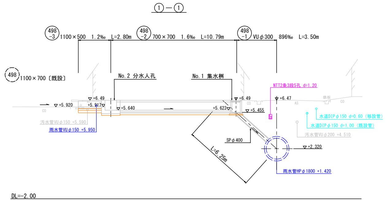
横断面図 S=1:50
