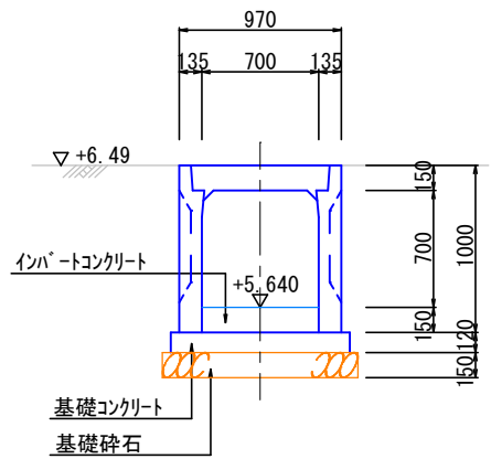
E-E断面
