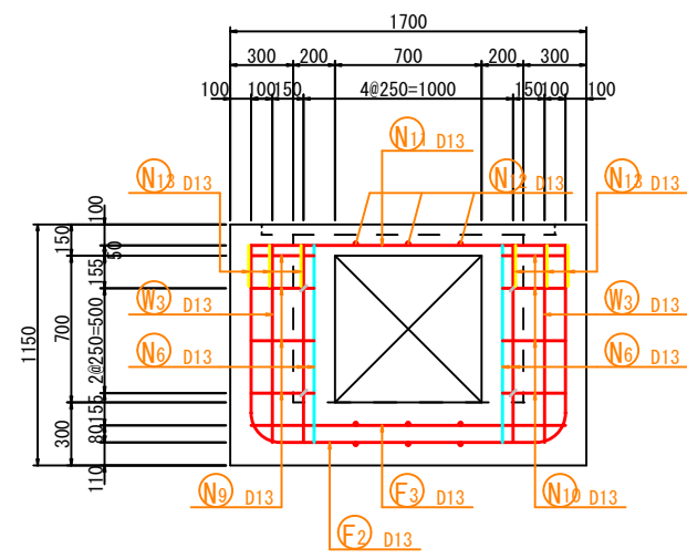
O - O (妻壁内面)
