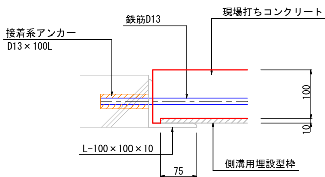
a部詳細図 S=1:4
