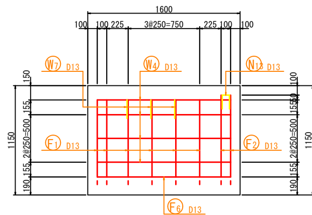
J - J (側壁外面)
