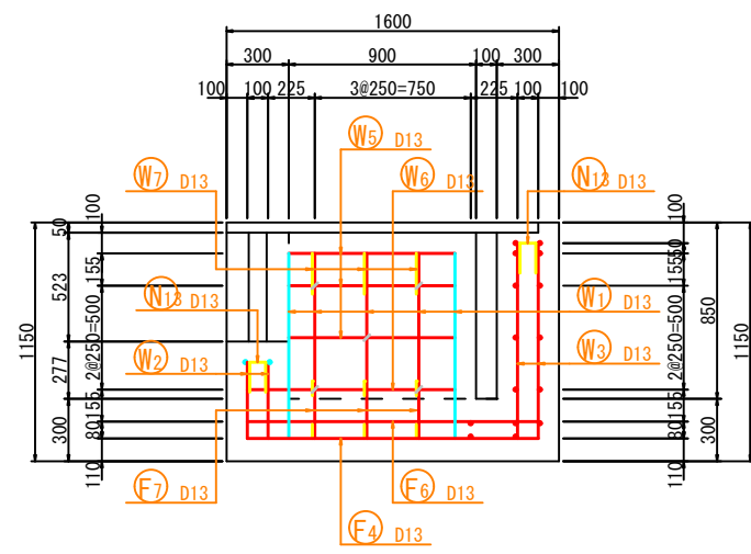
K - K (側壁内面)
