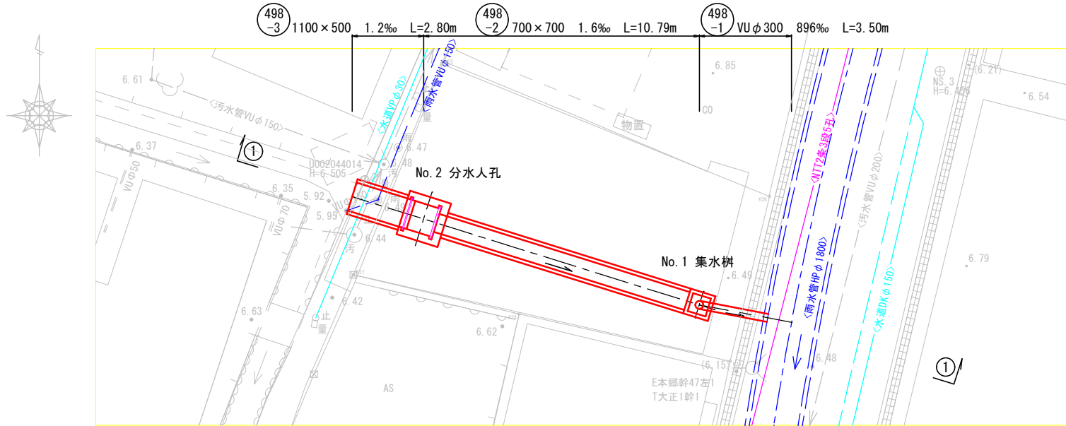
平面図 S=1:100
