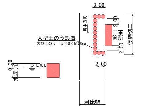
河川工事濁水対策標準断面
