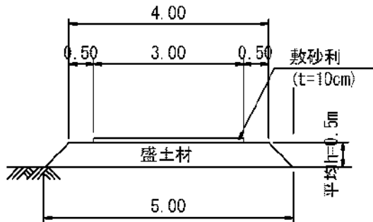
盛土タイプ
