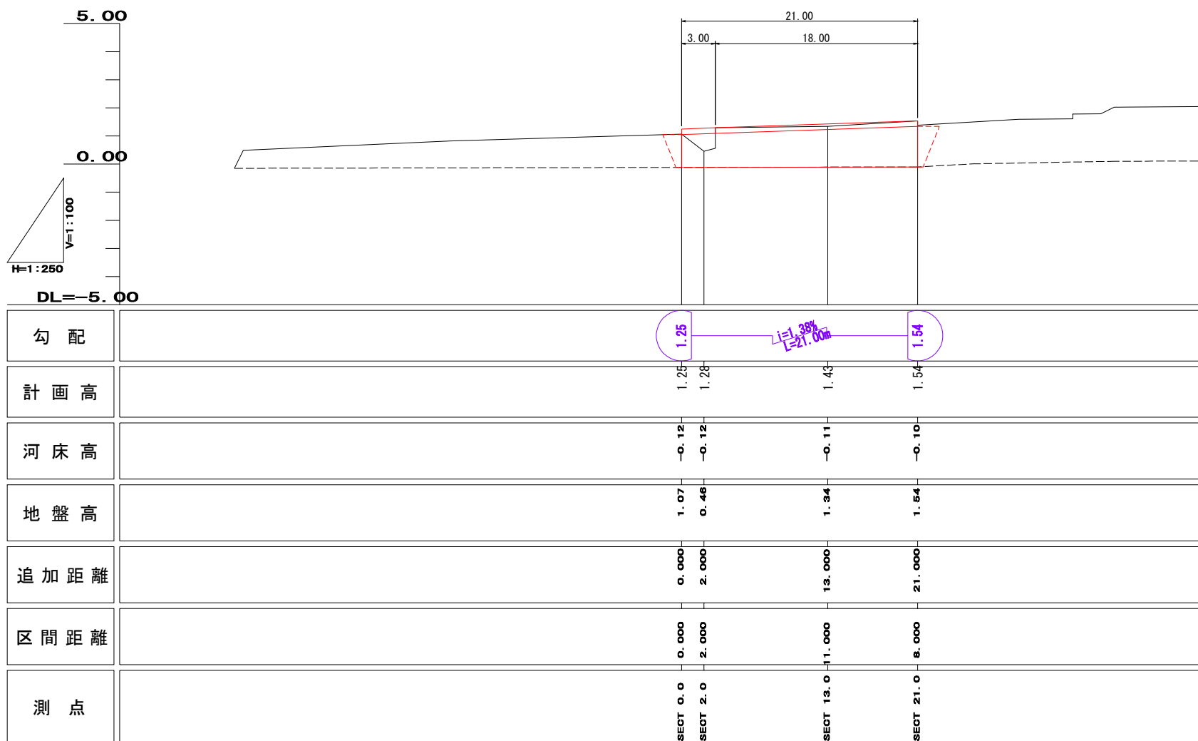
縦断図
