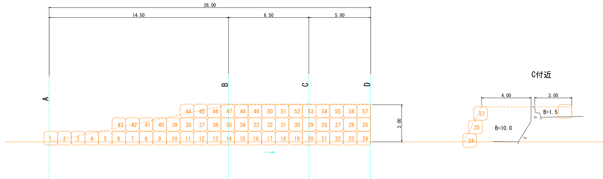
土のう展開図 S=1:100
