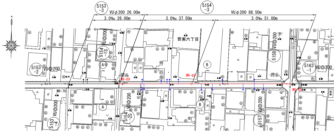
平面図 S=1/500
