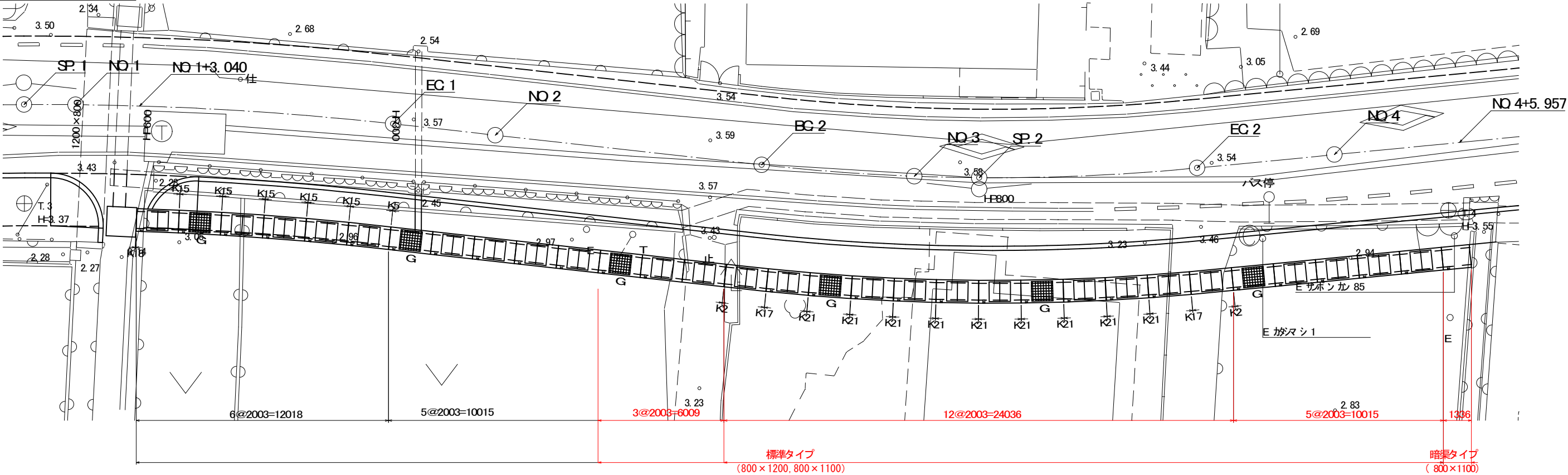
平面割付図 S=1/100
