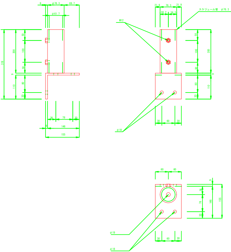
支柱径60.5mm用 (溶融亜鉛メッキ)
