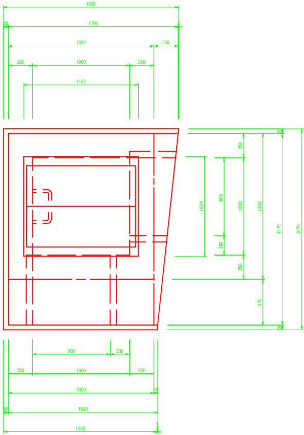
2号集水桝 S=1:20
