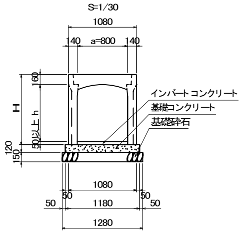
標準断面図
