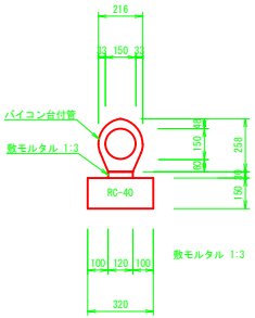
重圧管D150 S=1:20
