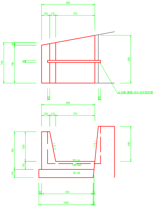
4号L型水路 S=1:20
