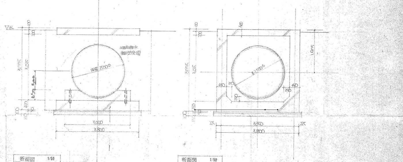
断面図 1/50
