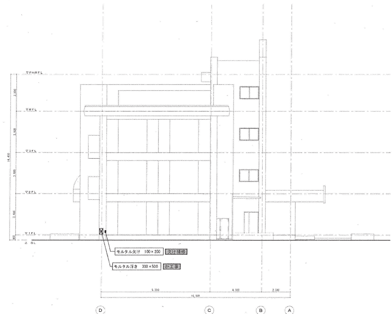
西面立面図 1/100
