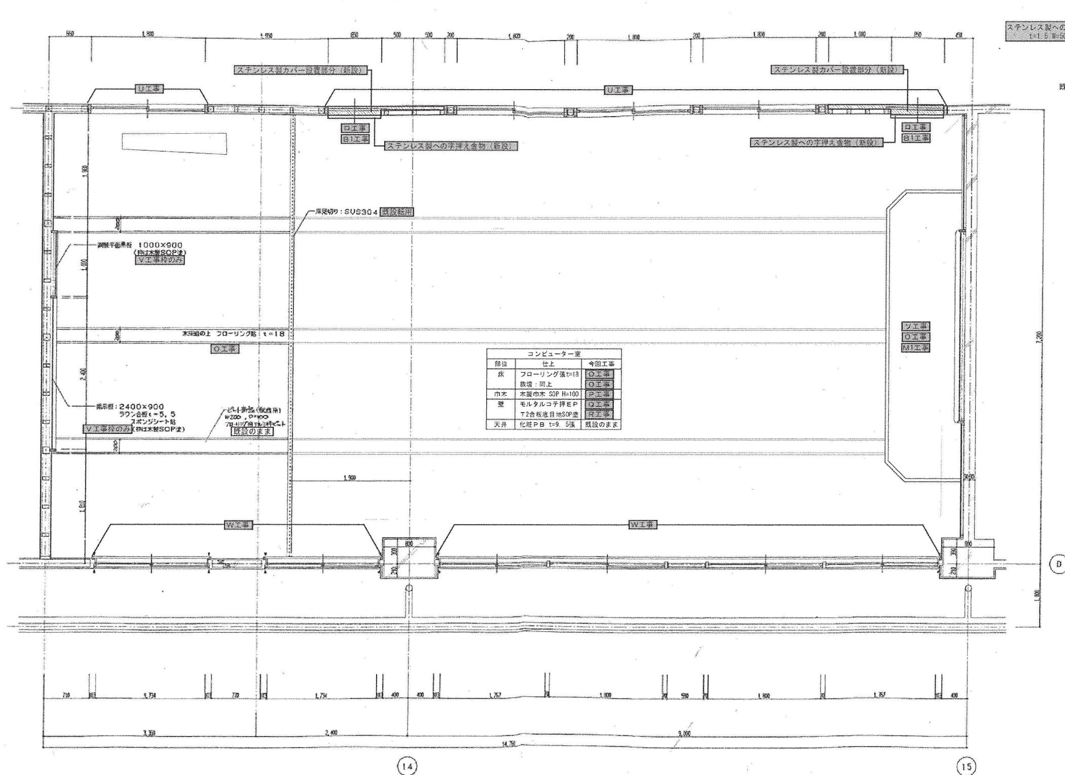
コンピュータ室 平面詳細図 1/30
