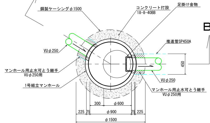
到達立坑部平面図 M-2-2
