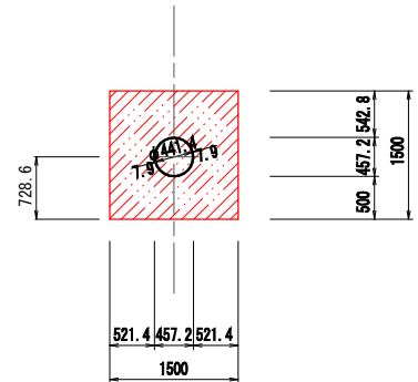
管路部断面
