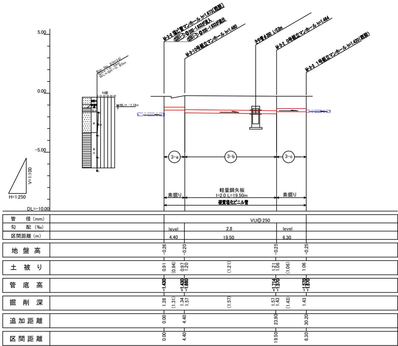
縦断面図 V=1:100 H=1:250
