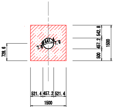
管路部断面
