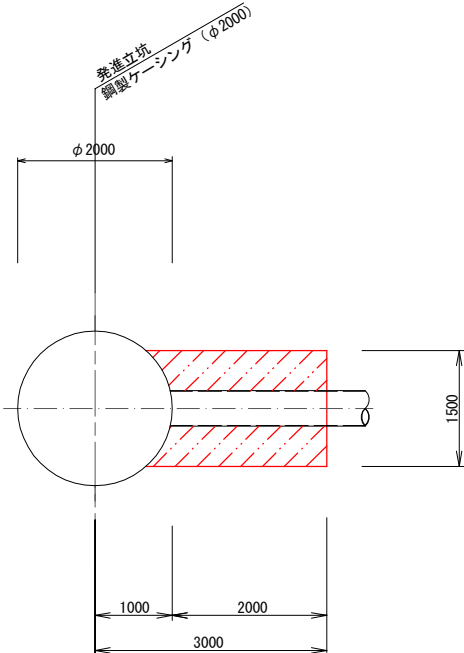
平面図
