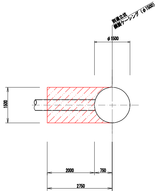
平面図
