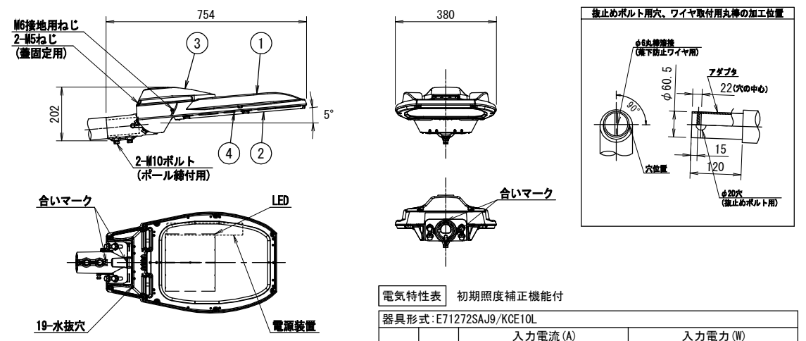
LED道路照明詳細図 S=1/10 E71272SAJ9/KCE10L (建電協形式: KCE100-2)
