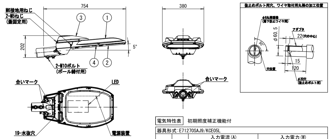
LED道路照明詳細図 S=1/10 E71270SAJ9/KCE05L (建電協形式: KCE050-2)
