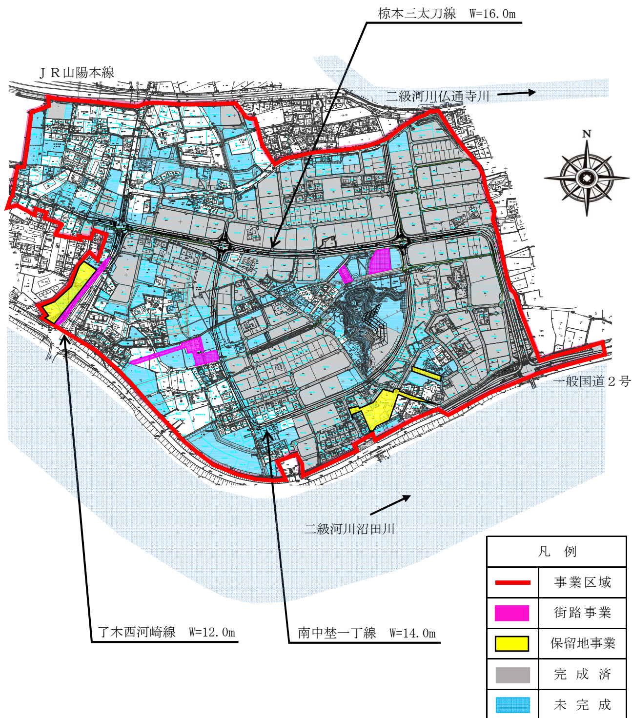
東本通土地区画整理事業平面図
