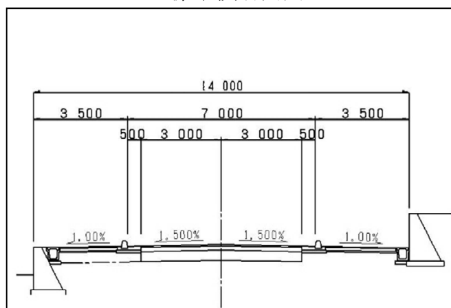
標準横断面図
