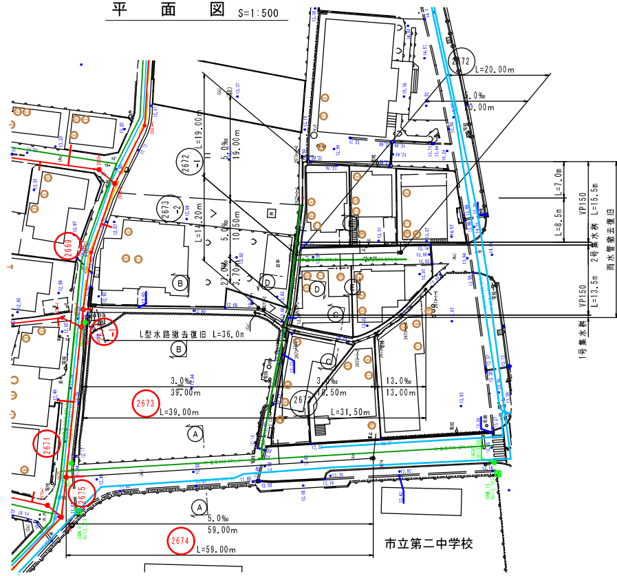
平面図 S=1:500
