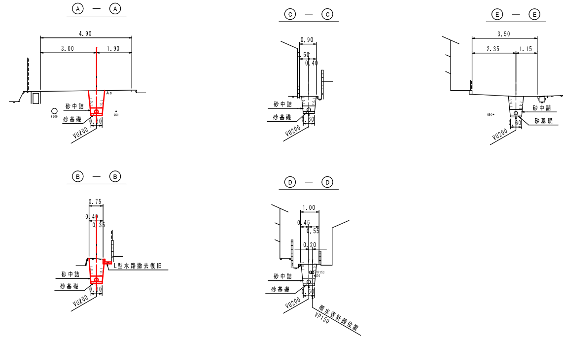
横断図 S=1:100
