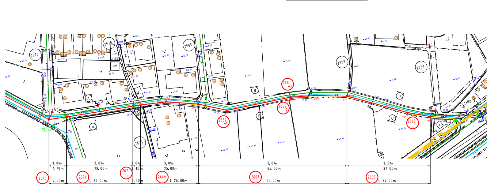
平面図 S=1:500
