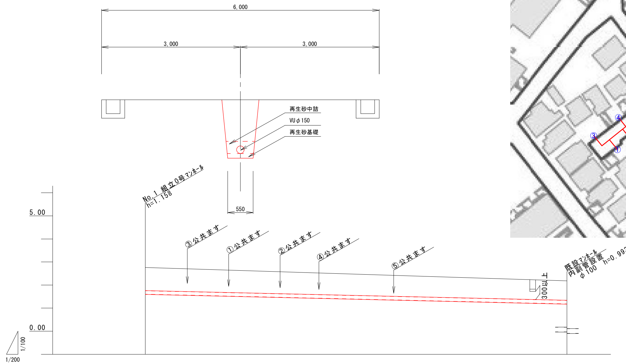
横断図 S=1/50
