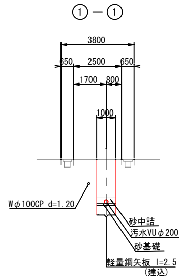
横断面図 S=1:100
