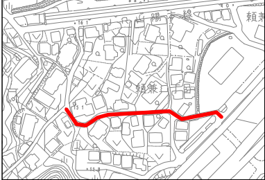
施工位置図 S=1/ 2,500
