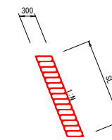
土のう積工(小口並べ)エ S=1:50
