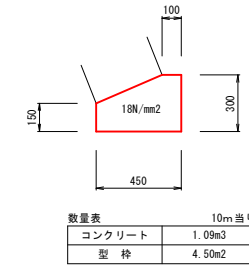
ブロック基礎 S=1:20
