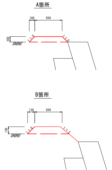
畦畔築立 S=1:20
