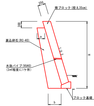
1号ブロック積擁壁 S=1:50 (A箇所)
