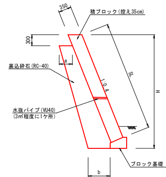
2号ブロック積擁壁 S=1:50 (B箇所)
