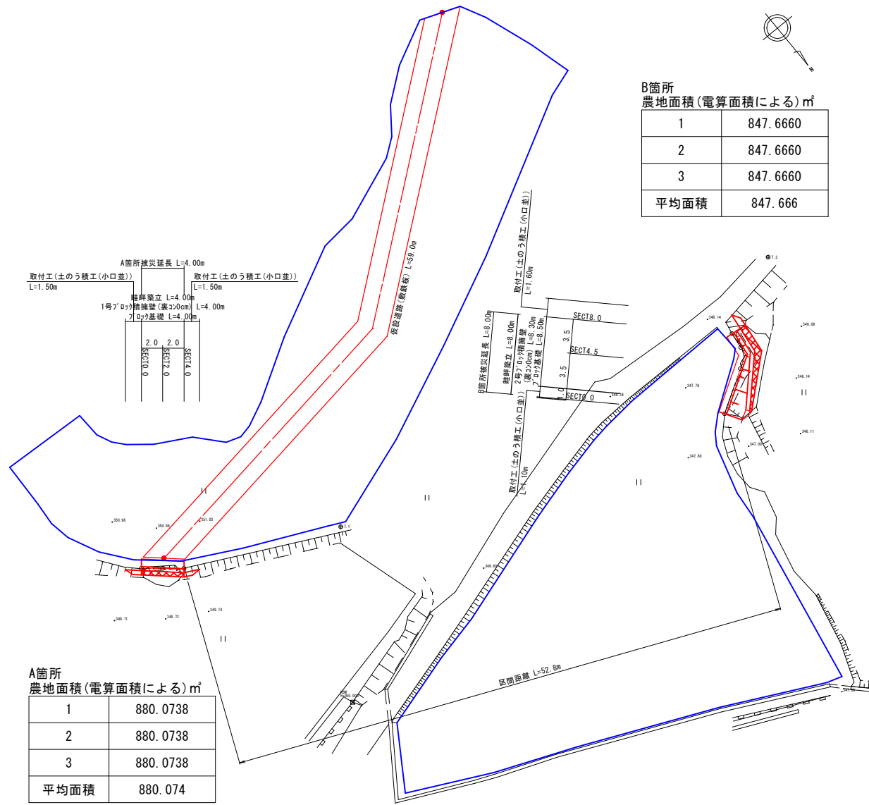
展開図 S=1:100
