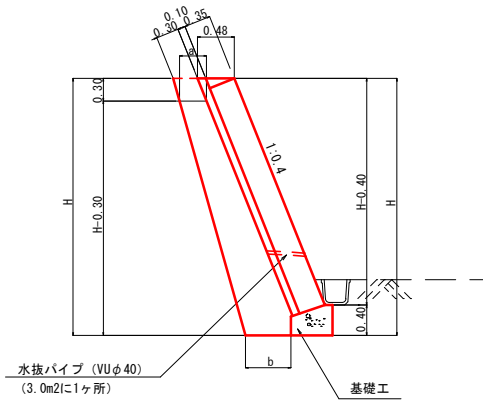
裏込砕石数量、寸法表(1:0.4)
