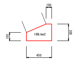
ブロック基礎 S=1:20 (A箇所)
