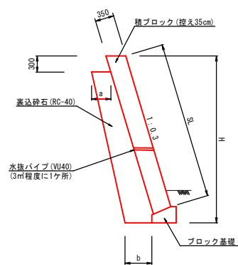
1号ブロック積擁壁 S=1:50 (A箇所)
