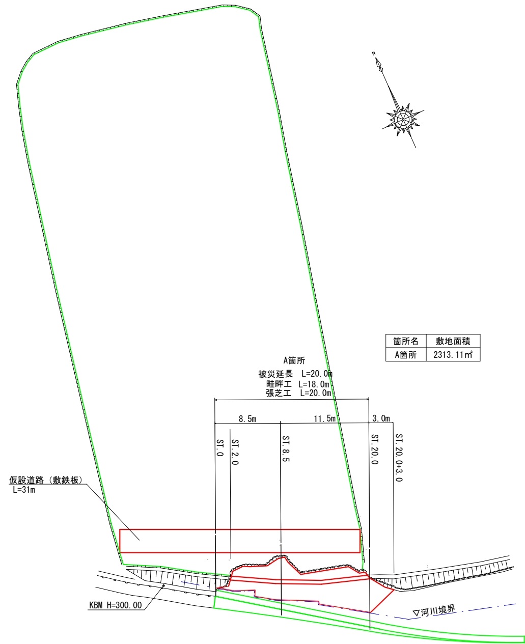
平面図 S=1:250
