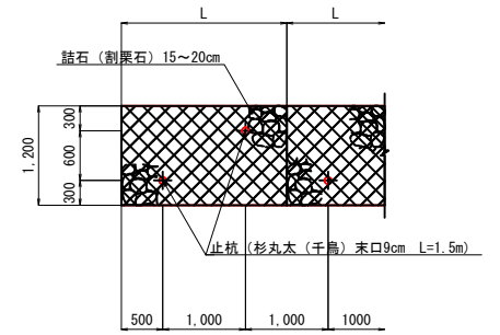
側面図 S=1:50
