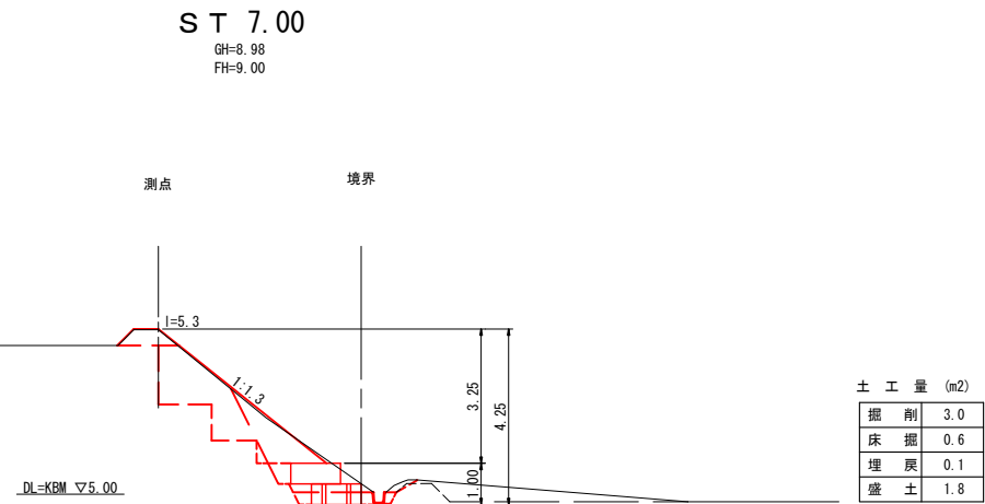
計画横断面図 S=1:100
