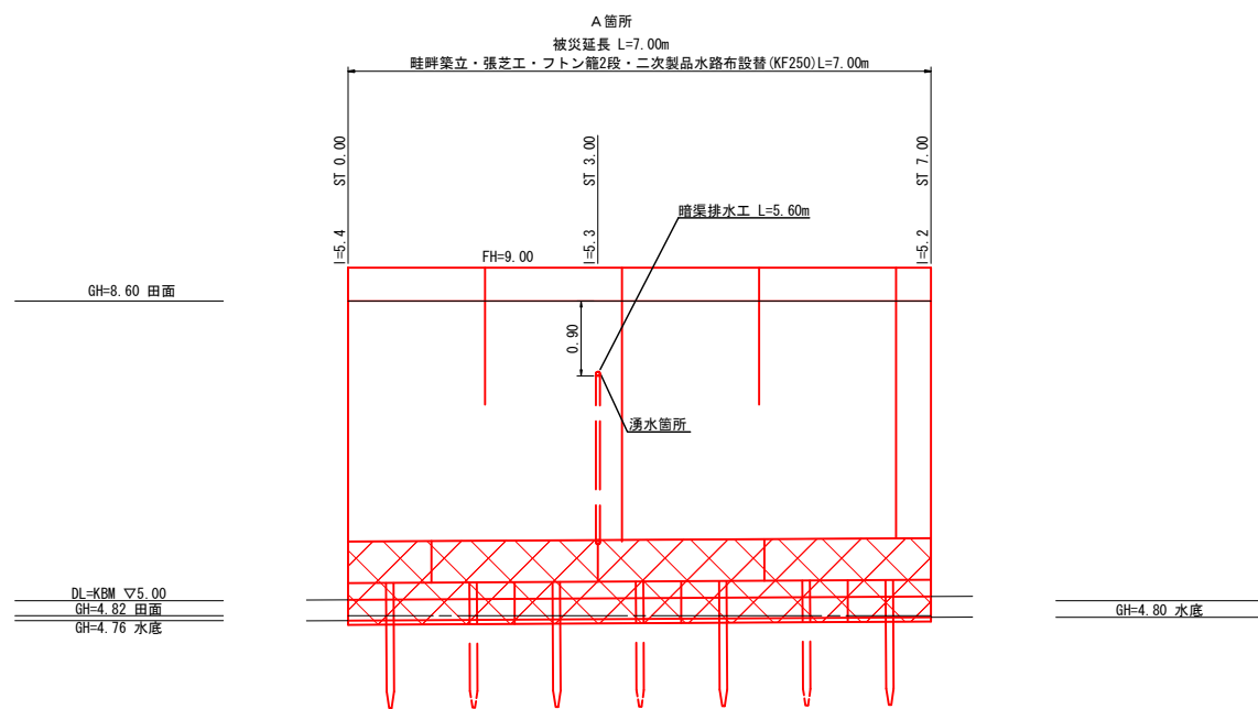
展開図 S=1:50
