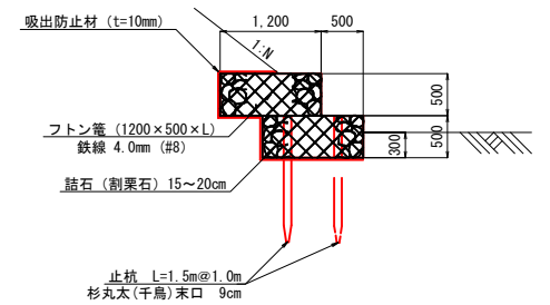
暗渠排水工 S=1:20
