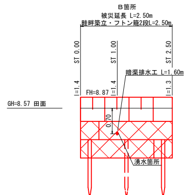
展開図 S=1:50
