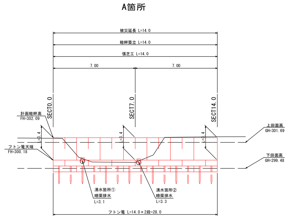
展開図 S=1:100
