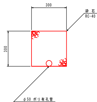
暗渠排水 縮尺=1:10
