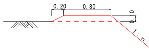
畦畔築立 S=1:20
