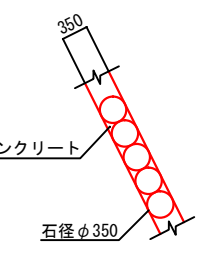
基礎工 S=1:20
