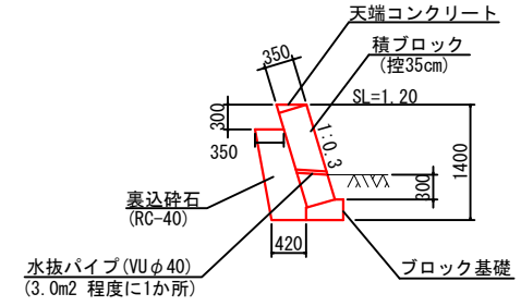
ブロック積擁壁 S=1:50
