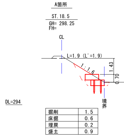
横断図 S=1:100
