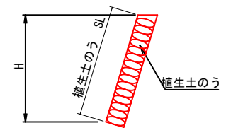
すりつけ工(練石積) S=1:50
