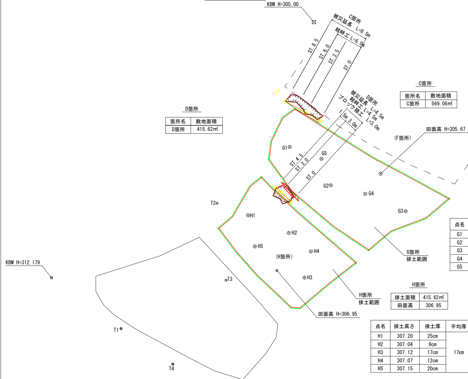
平面図 S=1:250
