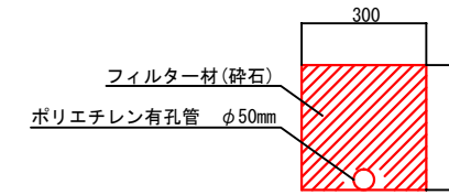
暗渠排水 S=1:10
