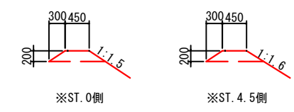
畦畔工 S=1:50
