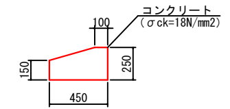
基礎工 S=1:20
