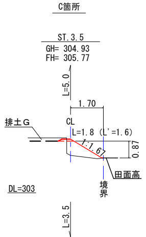
横断図 S=1:100
