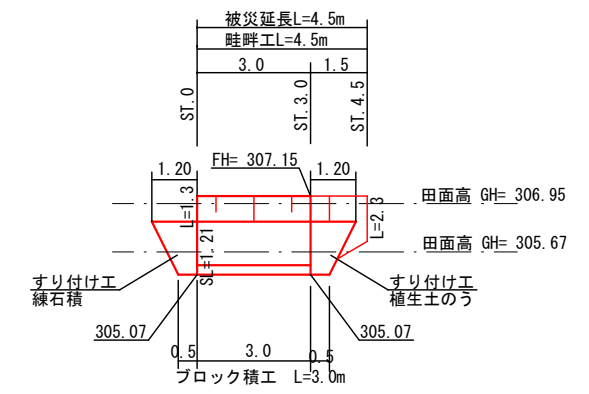
展開図 S=1:100
