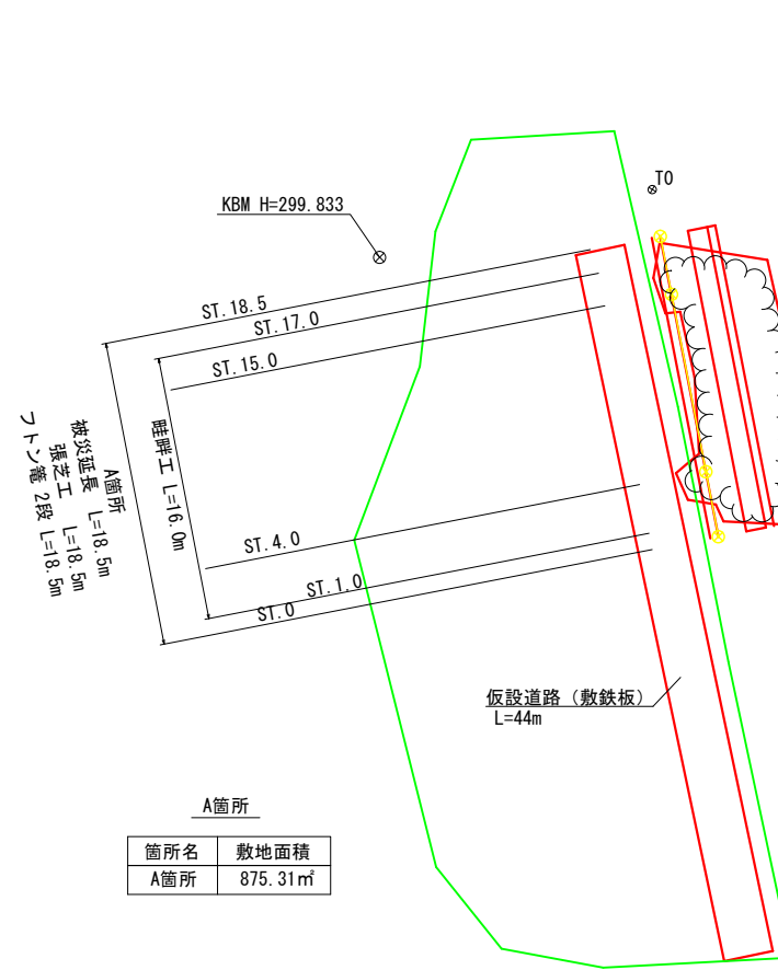
平面図 S=1:250
