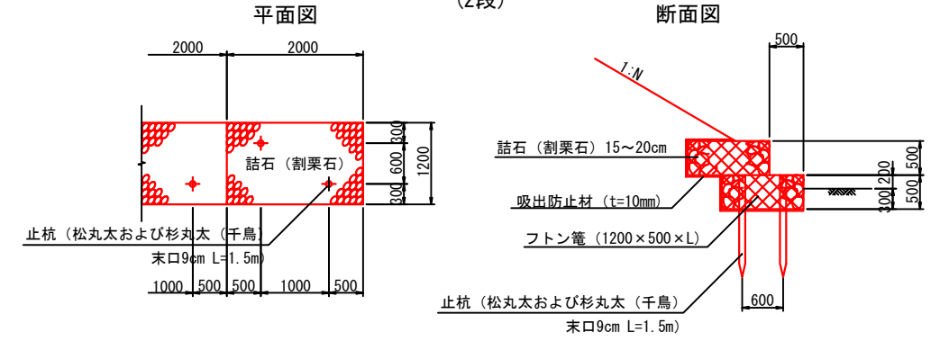
フトン籠 S=1:50 (2段)
