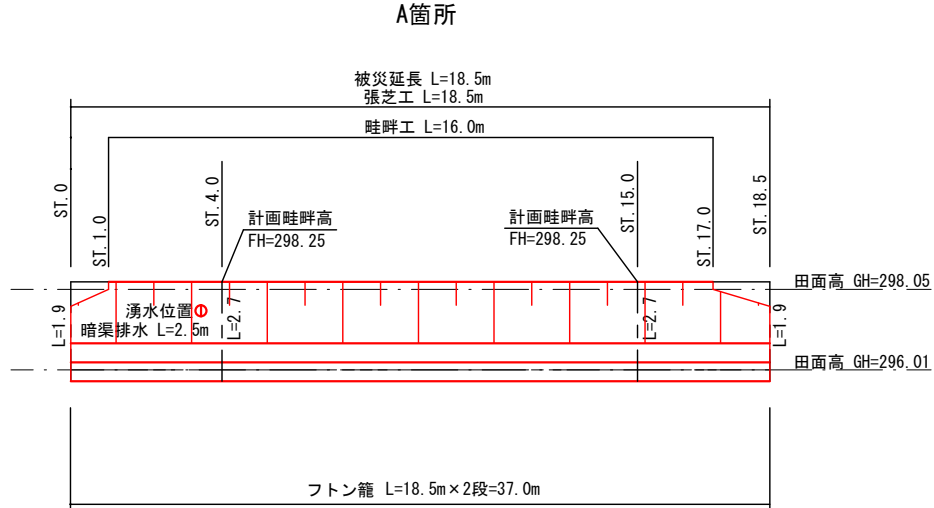
展開図 S=1:100
