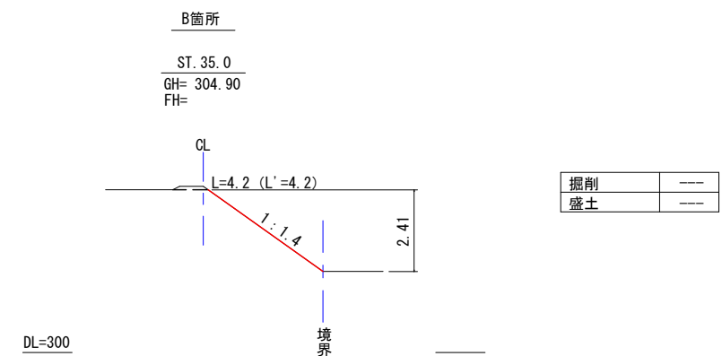
横断図 S=1:100
