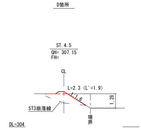
横断図 S=1:100
