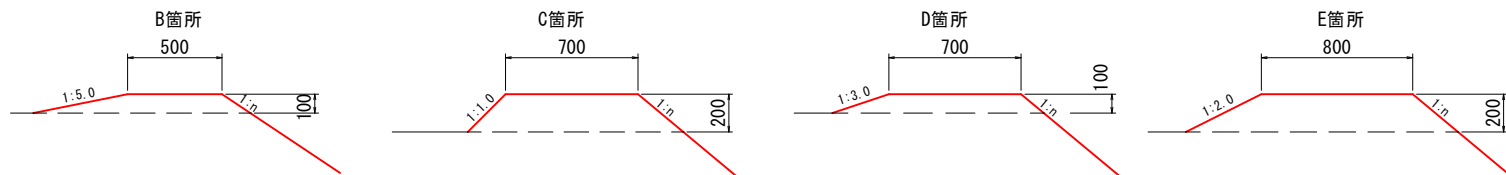
畦畔築立 S=1:20
