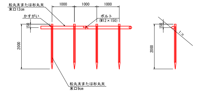
一本胴木 S=1:50
