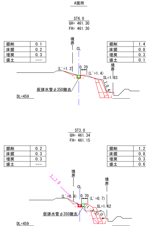
横断図 S=1:100
