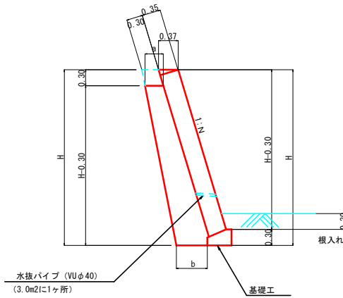
裏込砕石数量、寸法表 (1:0.4)
