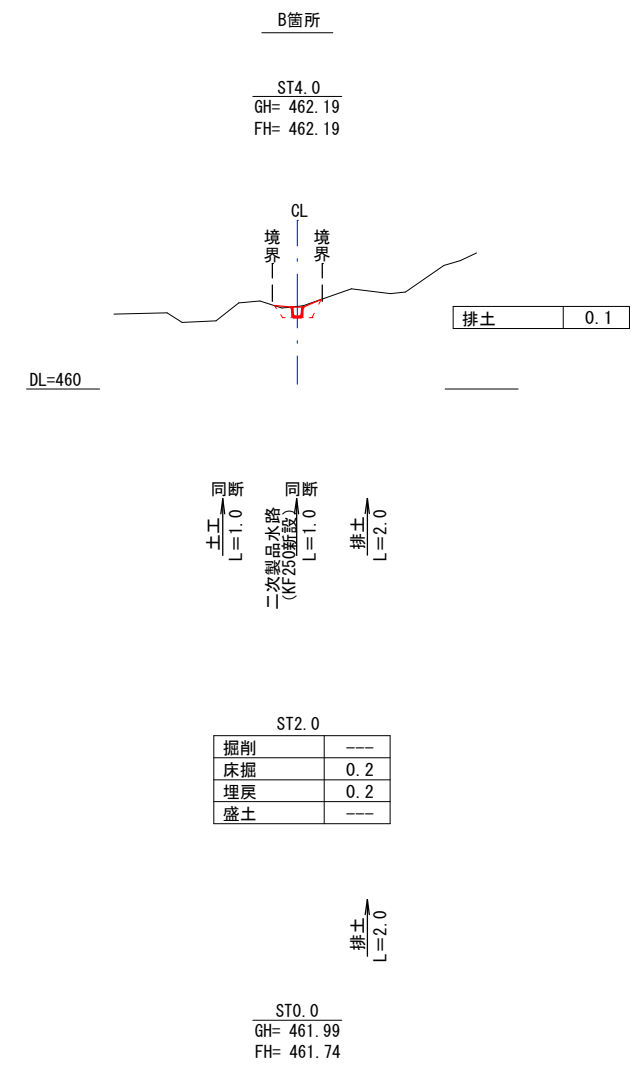
横断図 S=1:100
