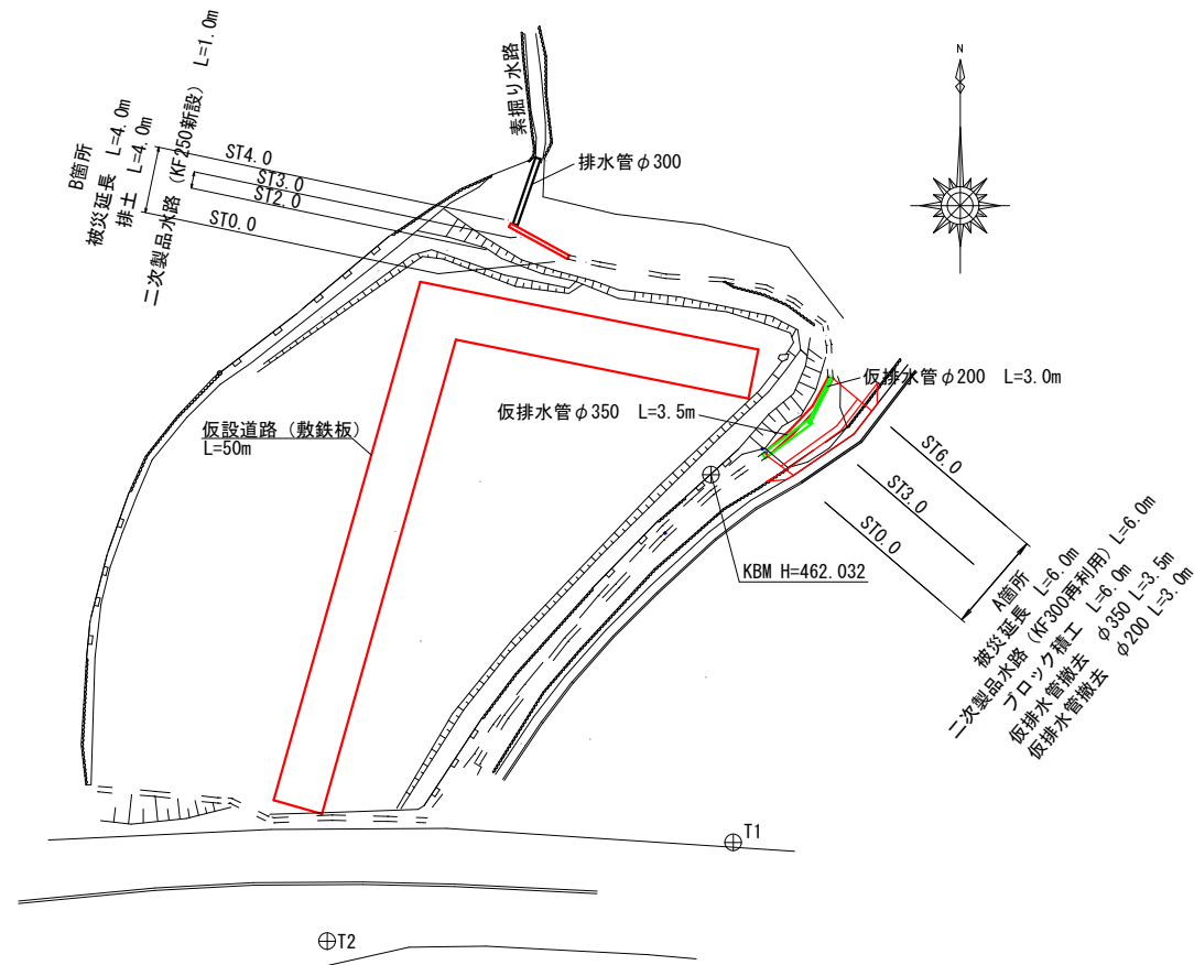
平面図 S=1:250
