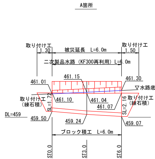
展開図 S=1:100
