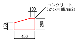
基礎工 S=1:20
