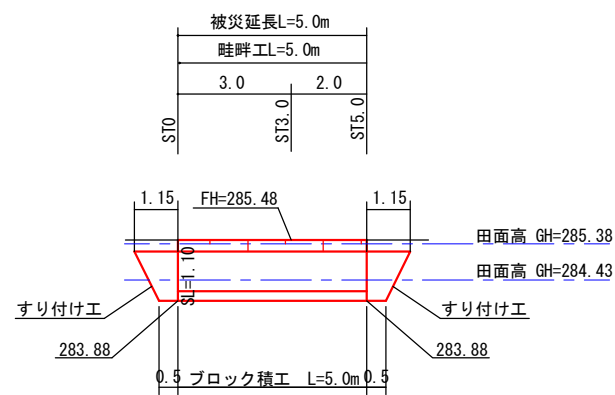
展開図 S=1:100 C箇所
