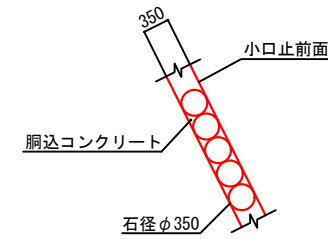
すりつけ工（練石積） S=1:50 (石材100%採取)
