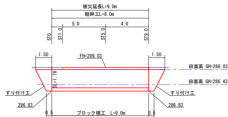
展開図 S=1:100 A箇所
