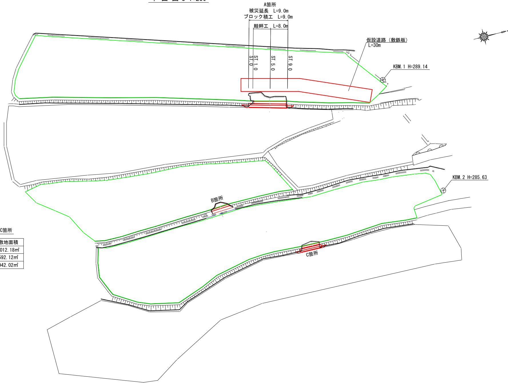
平面図 S=1:250
