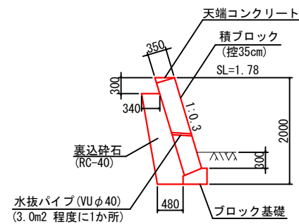
ブロック積擁壁 S=1:50
