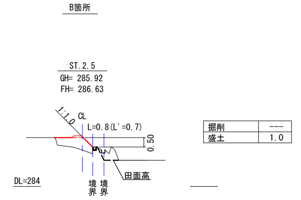
横断図 S=1:100
