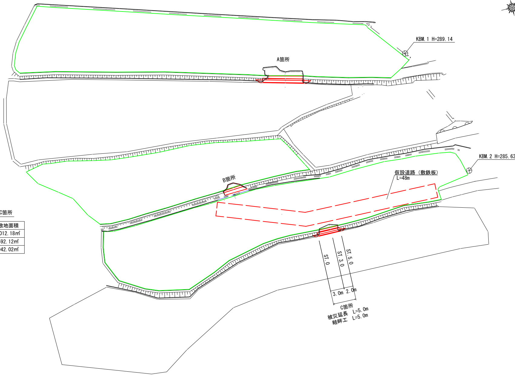
展開図 S=1:100 C箇所
