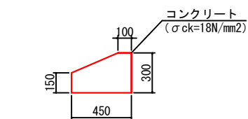
基礎工 S=1:20
