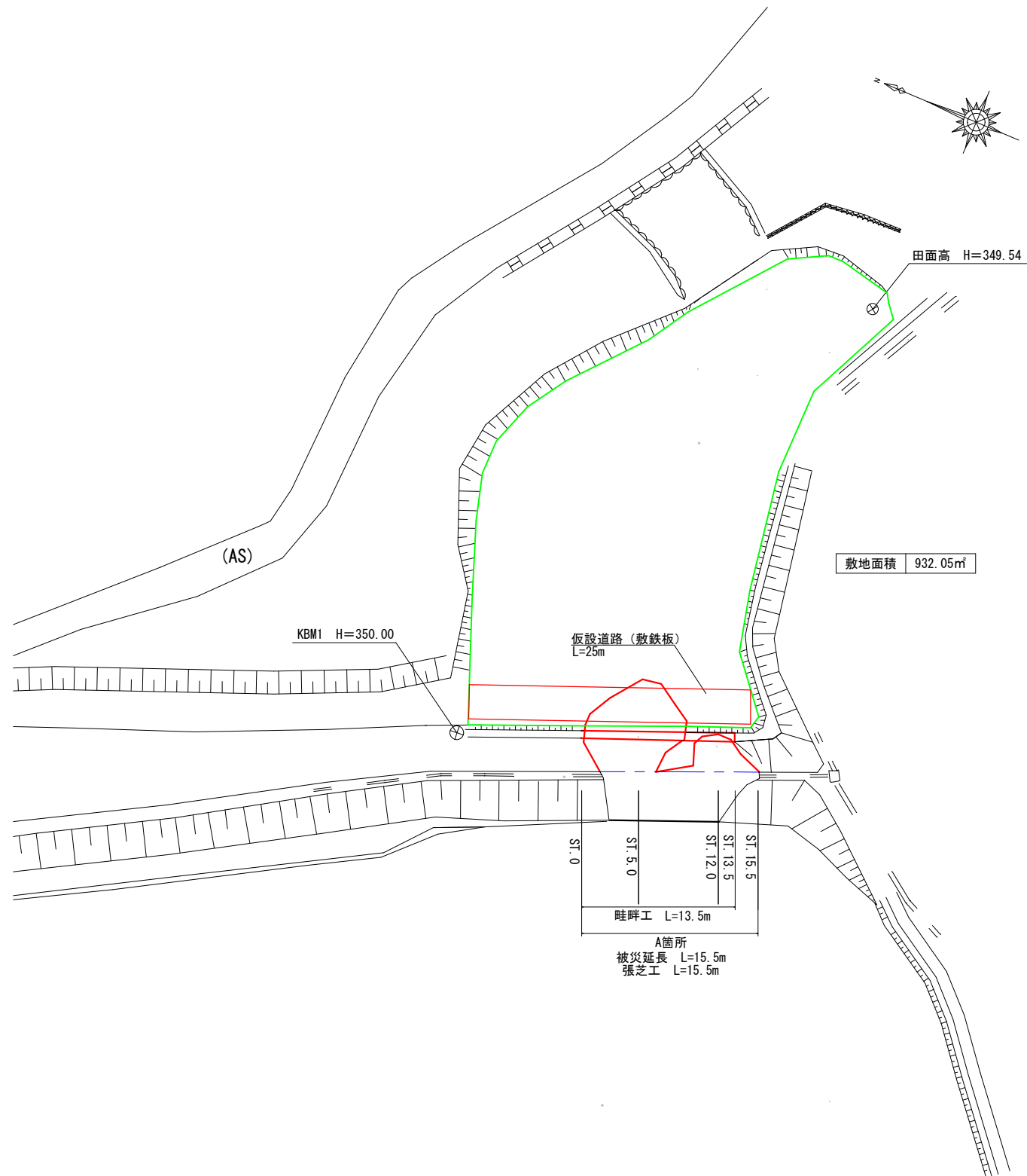
平面図 S=1:250
