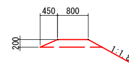
畦畔工 S=1:50
