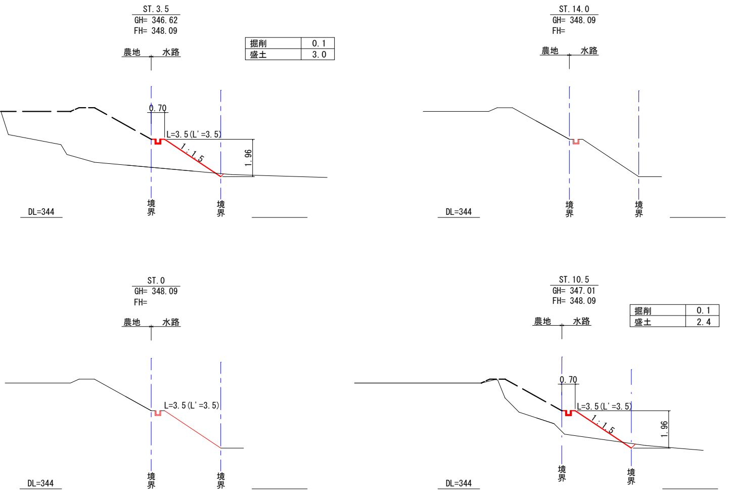
横断図 S=1:100
