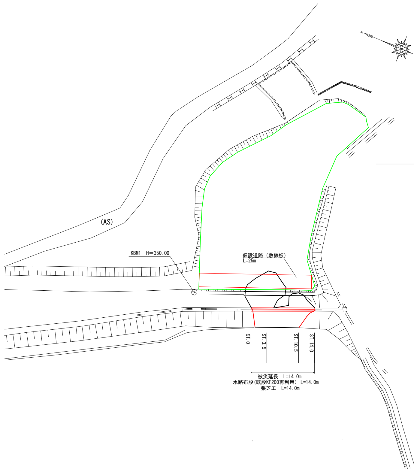
平面図 S=1:250
