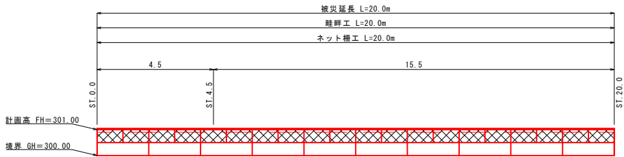
展開図 S = 1:100
