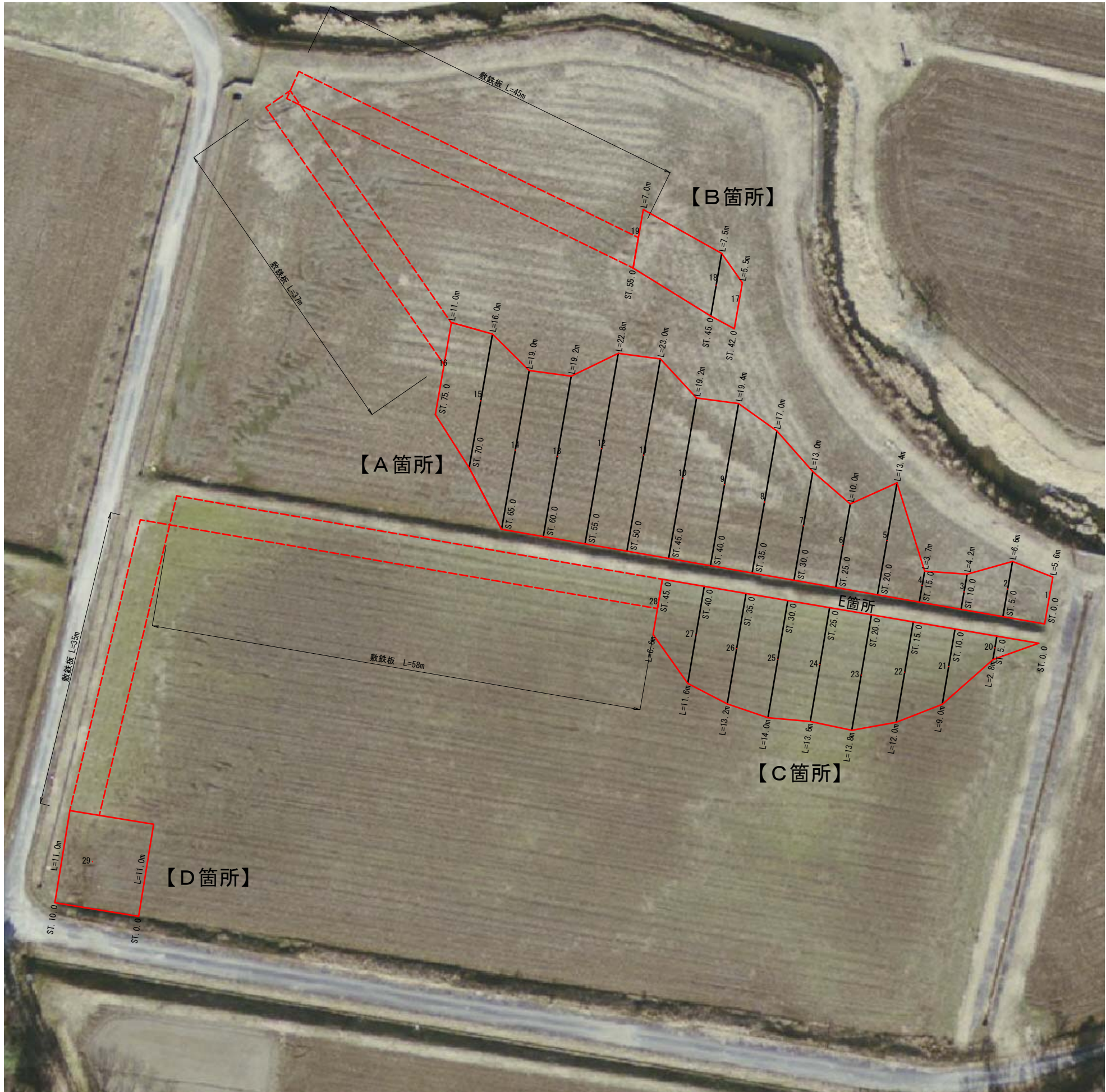
計画平面図 S=1:250
