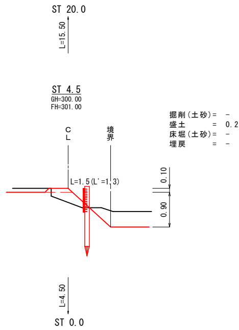
横断面図 S = 1:50
