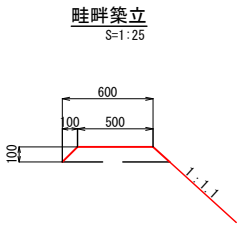
ネット柵工 S=1:50 H=500
