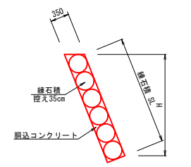
すりつけ工 S=1:50
