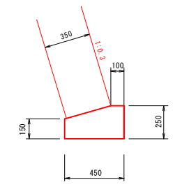
ブロック基礎 S=1:20
