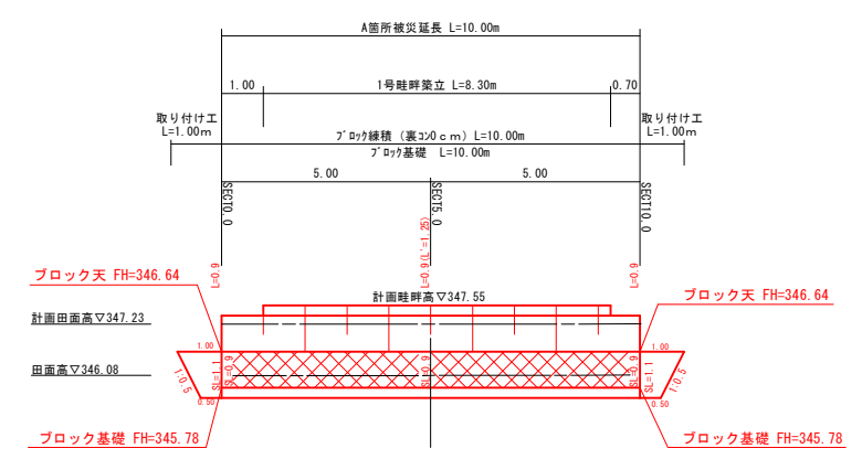
計画縦断面図
