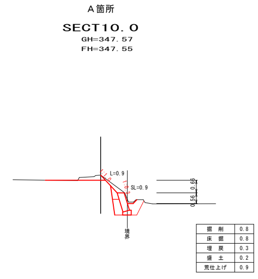
計画横断面図 S=1:100
