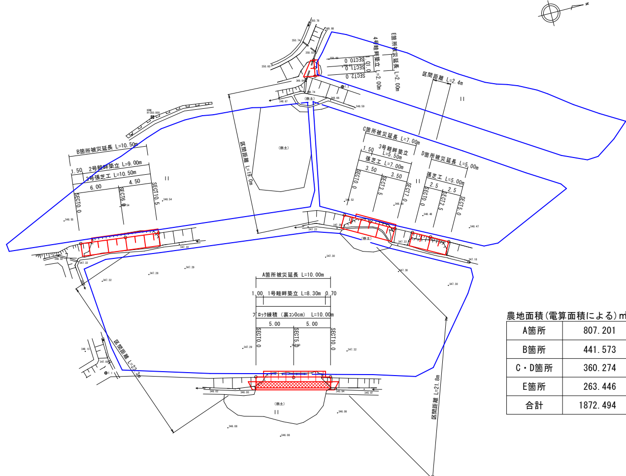
計画平面図 S=1:250
