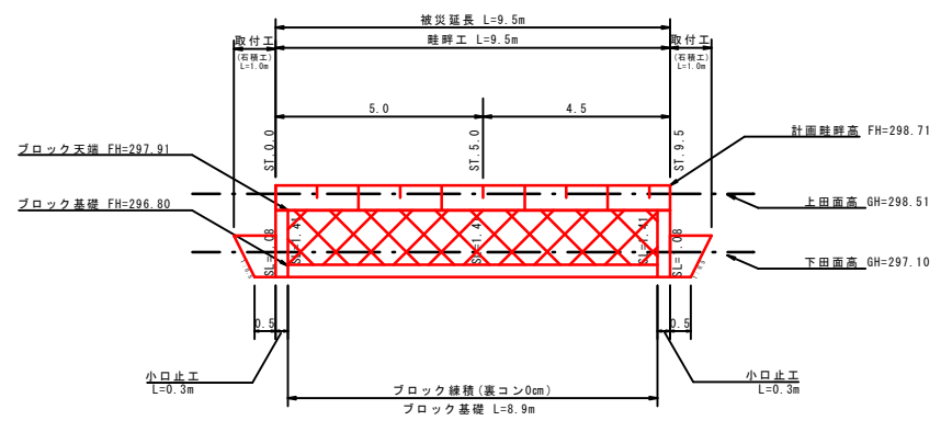
展開図 S=1:100
