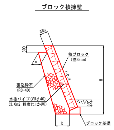
構造図 構造図
