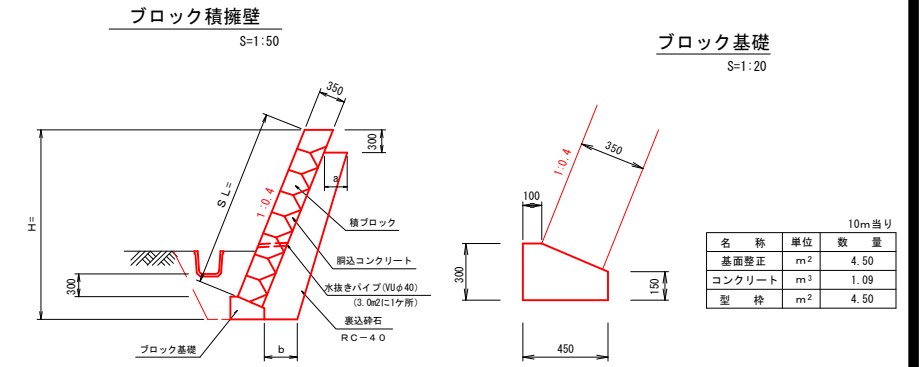
構造図
