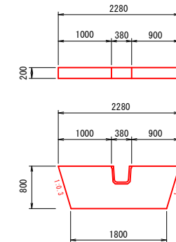
2号止水壁 S=1:50
