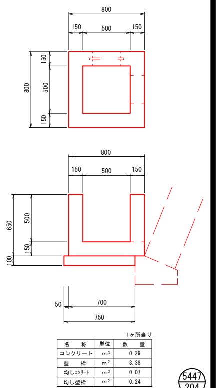
集水枡 S=1:20
