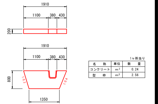
集水枡 S=1:20
