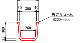
KF300 S=1:20
