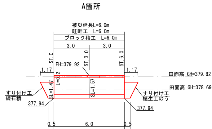
展開図 S=1:100
