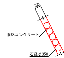
すりつけ工(練石積) S=1:50
