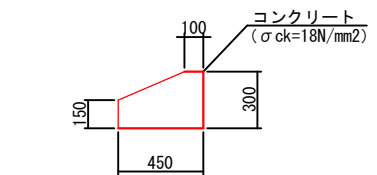
基礎工 S=1:20
