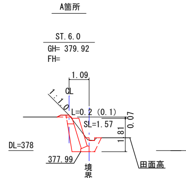
横断図 S=1:100
