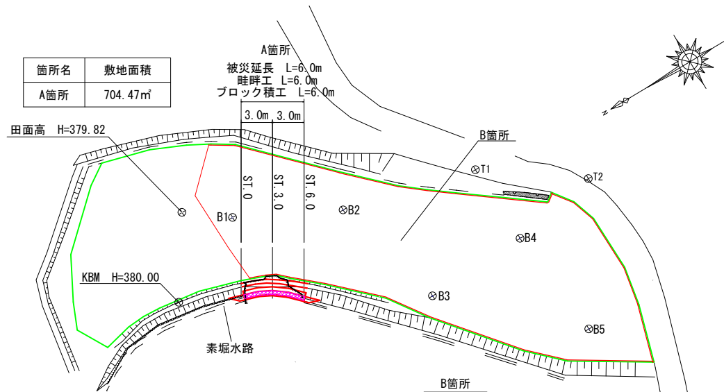
平面図 S=1:250
