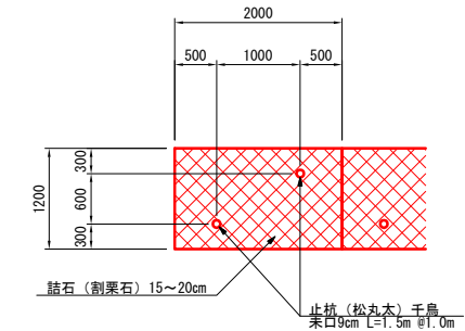
フトン管 S=1:50
