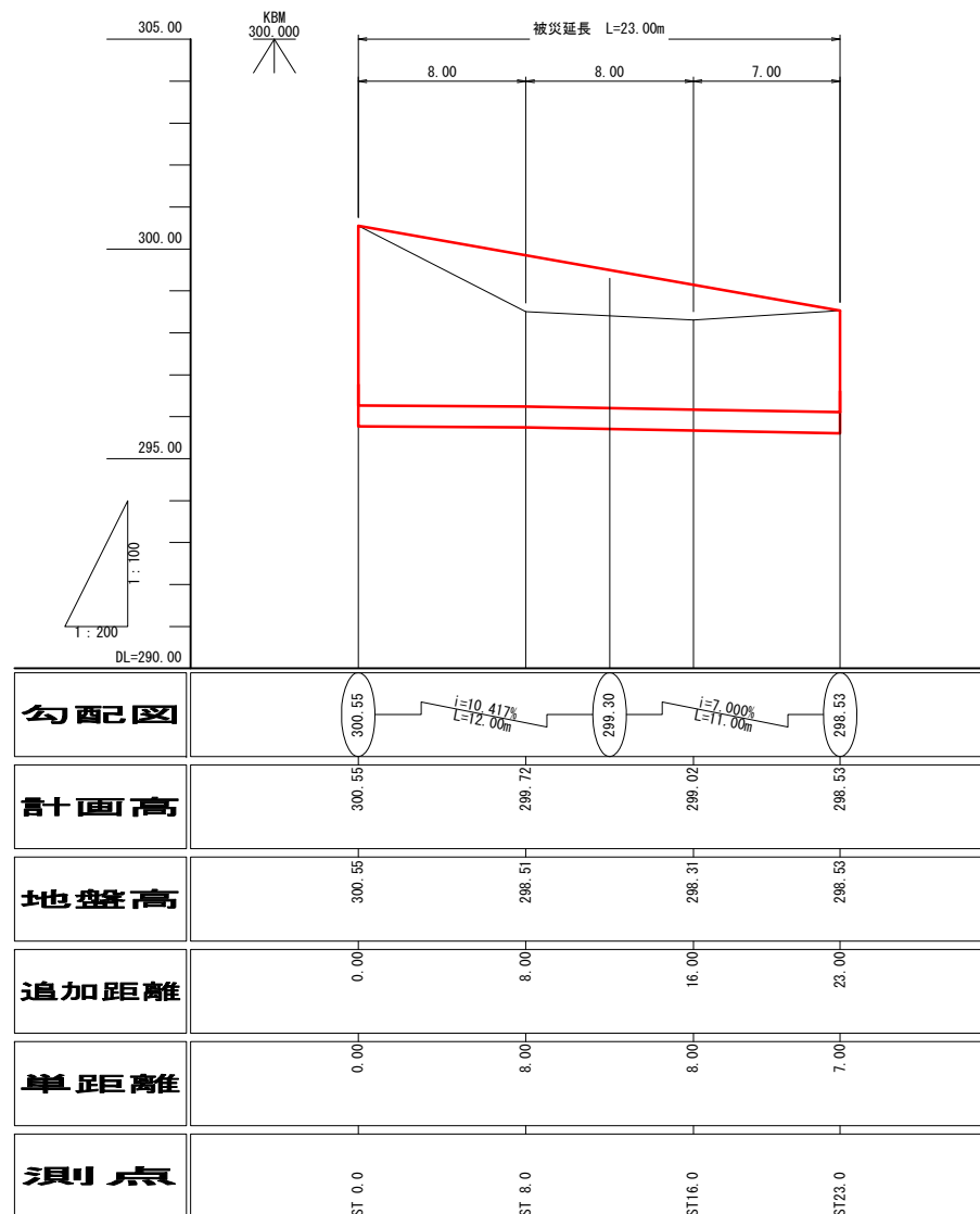
縦断面 V=1:100 H=1:200
