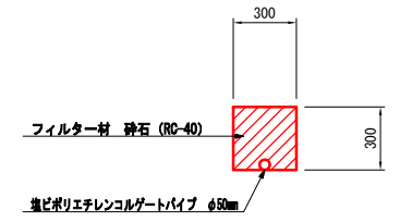
暗渠排水 S=1:20
