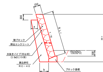
ブロック積擁壁 S=1:50
