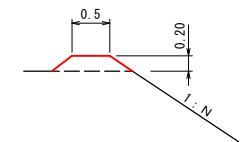
陸畔築立 S=1:50
