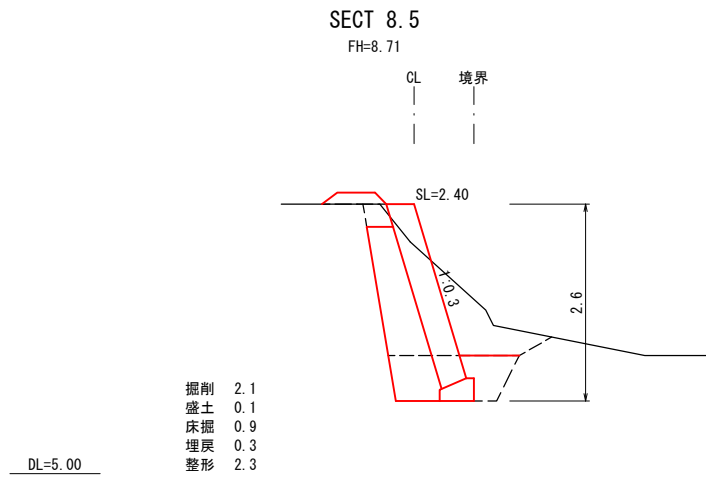
計画横断面 S=1:50
