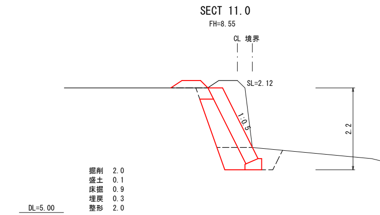
計画横断面 S=1:50
