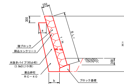
ブロック積擁壁 S=1:50
