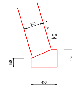
ブロック基礎 S=1:20
