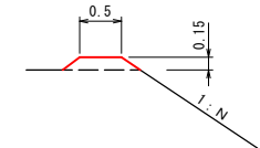
畦畔築立 S=1:50
