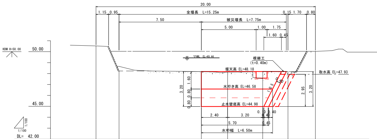
計画縦断面図 V=1:100 H=1:100
