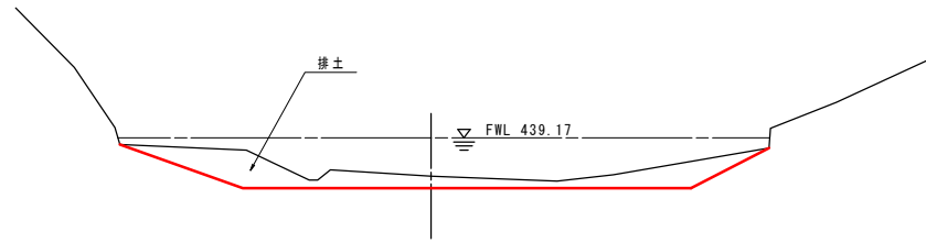
標準断面図 S=1:100
