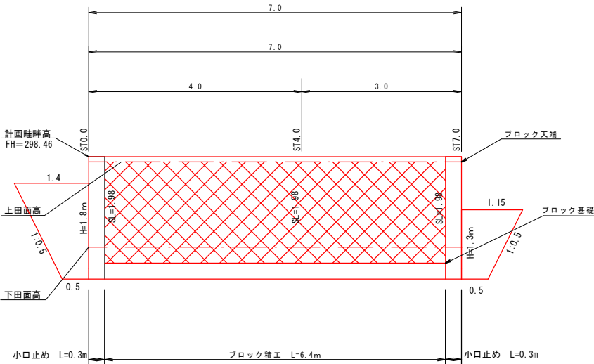
展開図 S = 1:50
