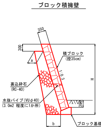
構造図
