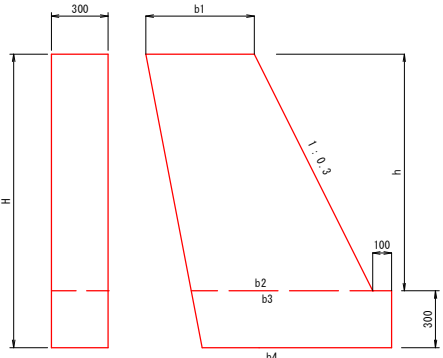
小口止工 S=1:20
