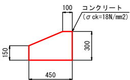
ブロック基礎 S = 1:20
