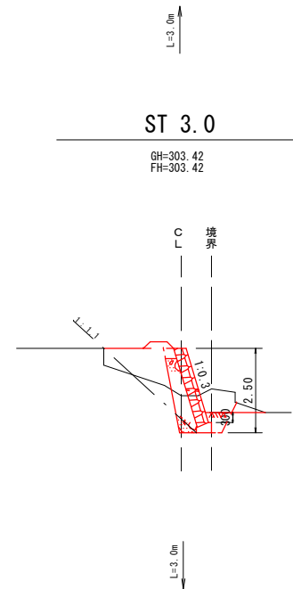
横断面図 S=1:100
