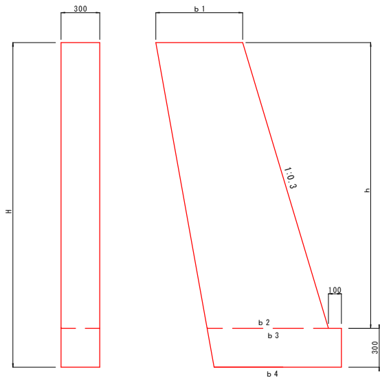
小口止工 S=1:20
