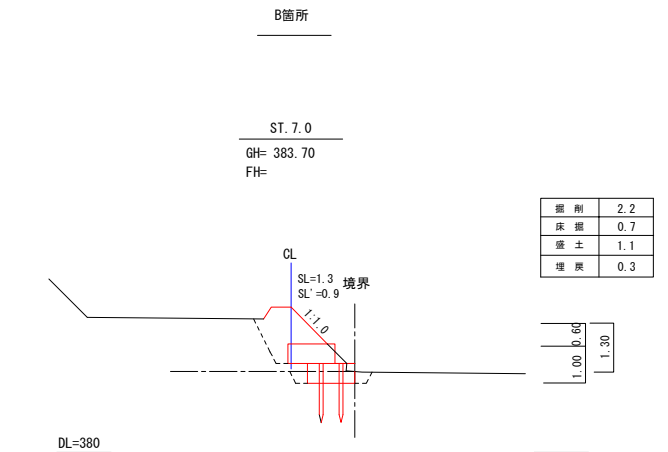
横断図 S=1:100
