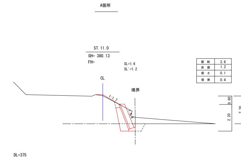
横断図 S=1:100
