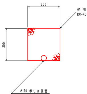
暗渠排水
