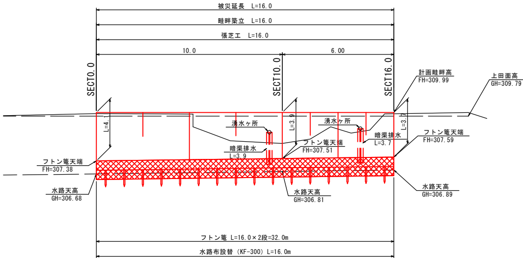
展開図 S=1:100
