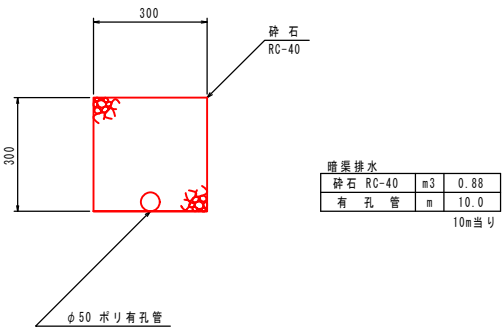
暗渠排水
