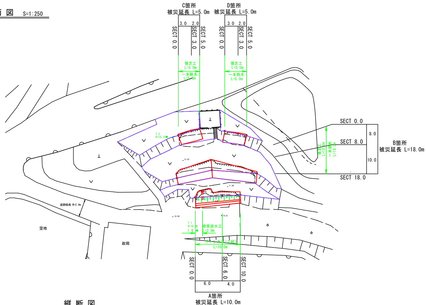
縦断図
