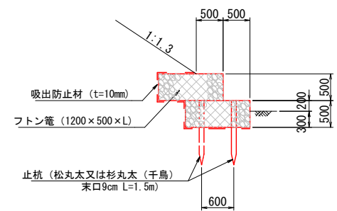
断面図
