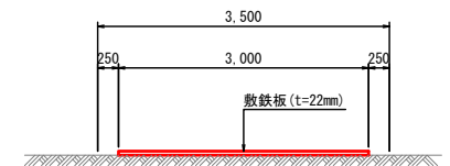
仮設道路 S=1:50
