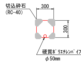
畦畔工 S=1:20
