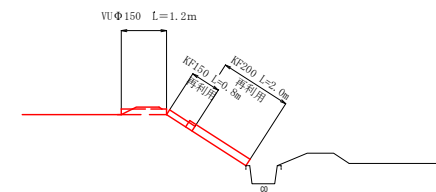
田面排水 S=1:100
