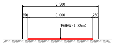
仮設道路 S=1:50
