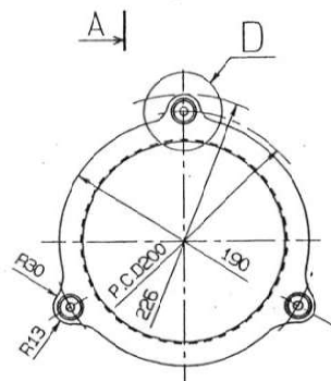
矢視A-A
