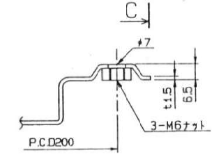
1:1 D詳細
