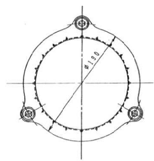
A-矢視
