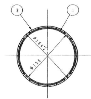
B-断面
