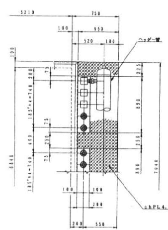
A部詳細
