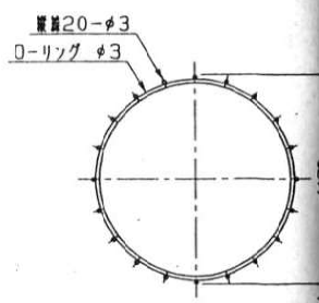
断面B-B
