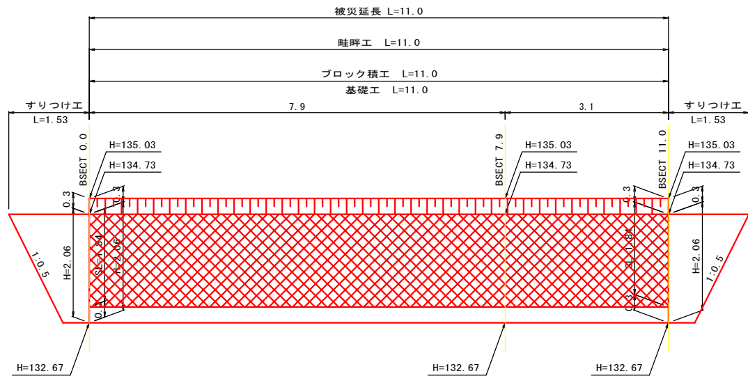
展開図 S=1:50
