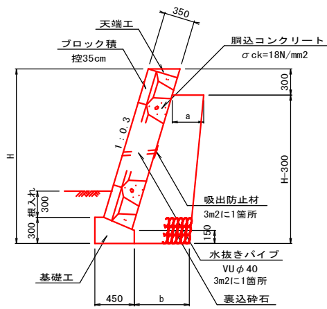
ブロック積擁壁 S=1:30
