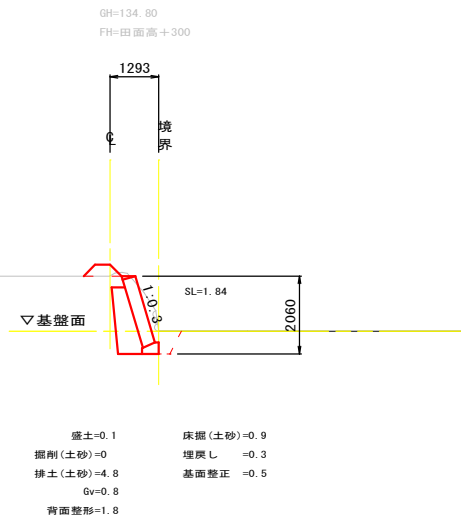
D=7.90 BSECT 0.00
