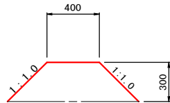
畦畔工 S=1:20
