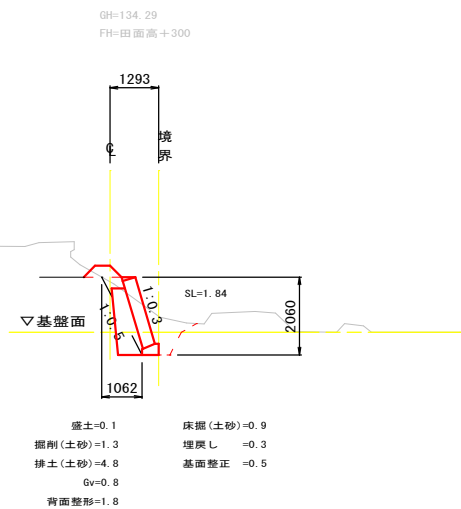
D=7.90 BSECT 0.00
