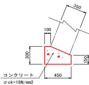
基礎工 S=1:20
