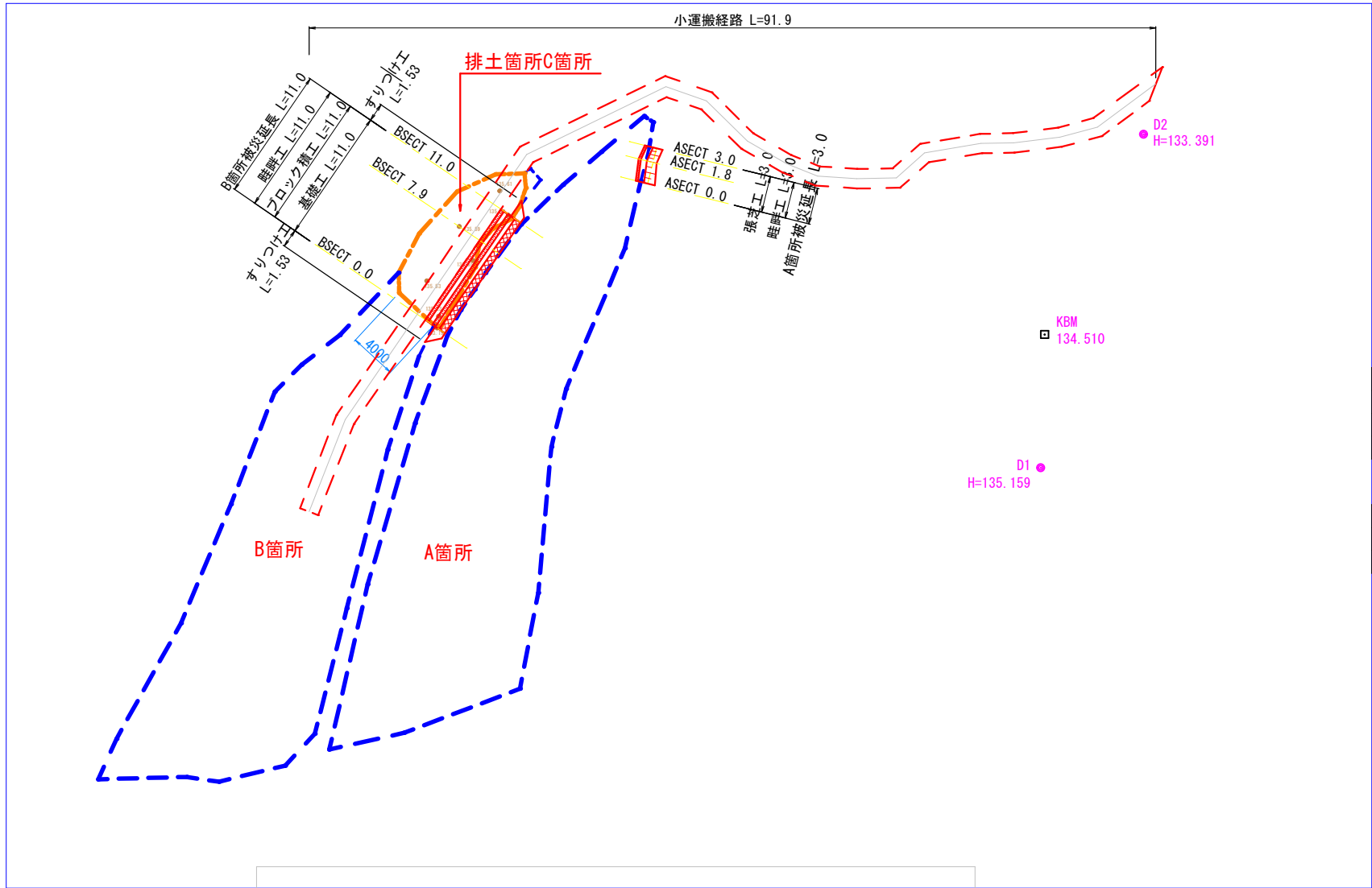
排土C箇所詳細図 S=1:100
