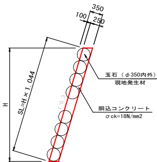
すりつけ工 S=1:50
